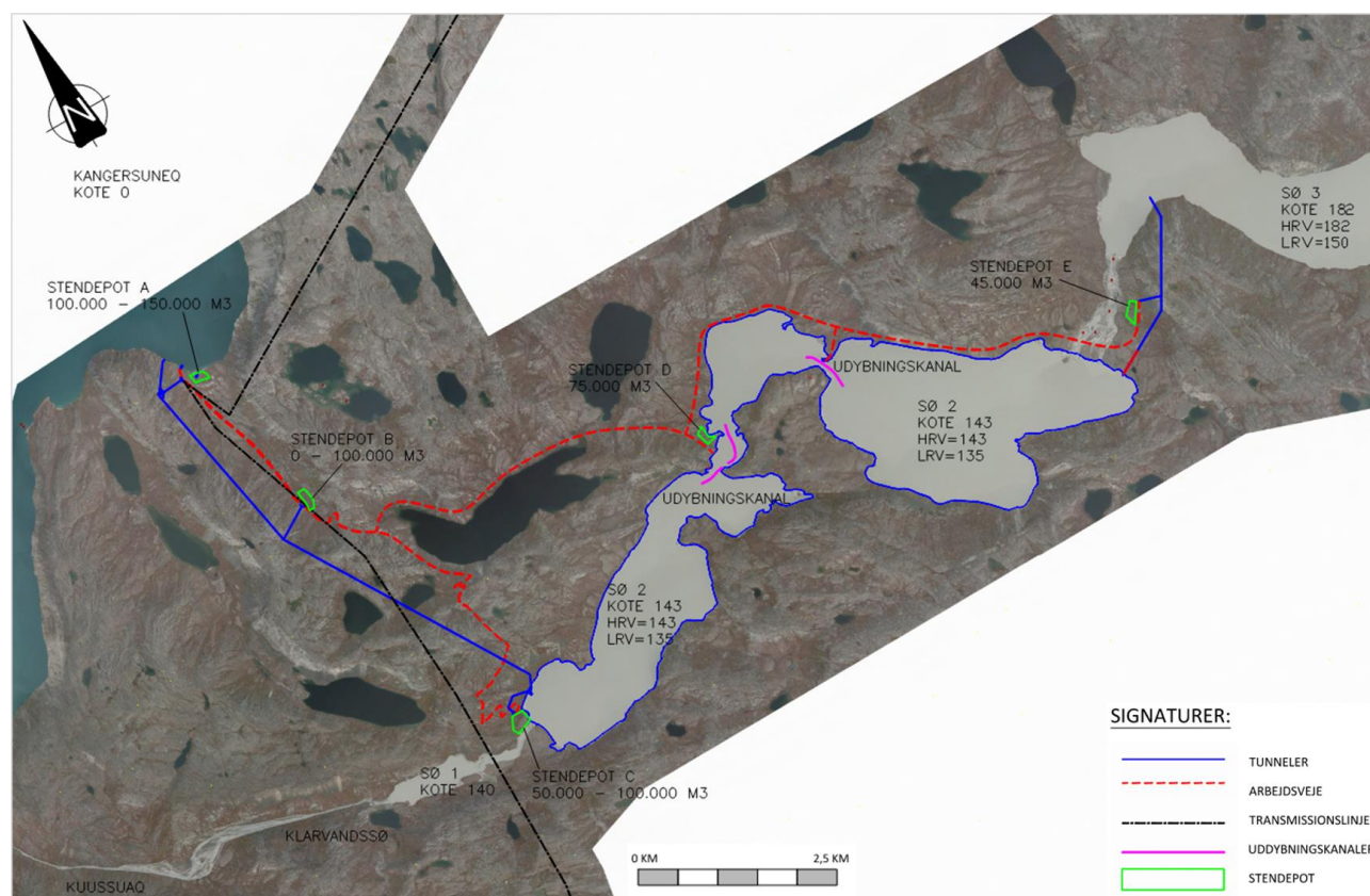
Takussutissiaq 57: Qaartiternerlukunik inissiiviit inissinneri.
