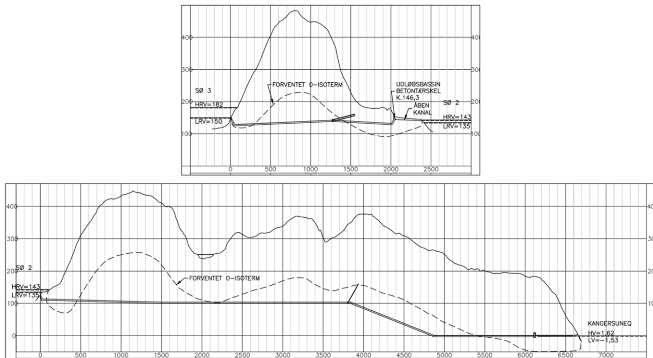
Takussutissiaq 45: Sulluliap kuutsitsiviup aamma sulluliat kuuffiit takissusiisa sanimut isigineqarnerat
