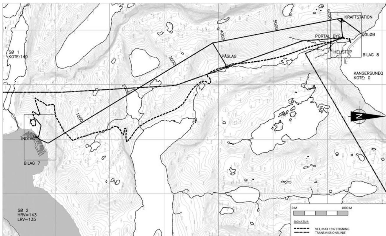
Takussutissiaq 44: Sullup tatsimut kuuffiup ingerlanera
