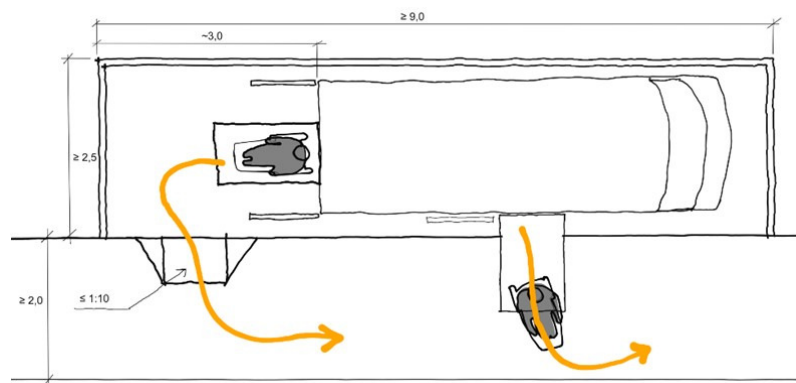
Figur 3: Eksempel på afsætningsplads eller parkeringsplads langs kantsten til kassevogn eller minibus med lift bagpå eller i siden.
