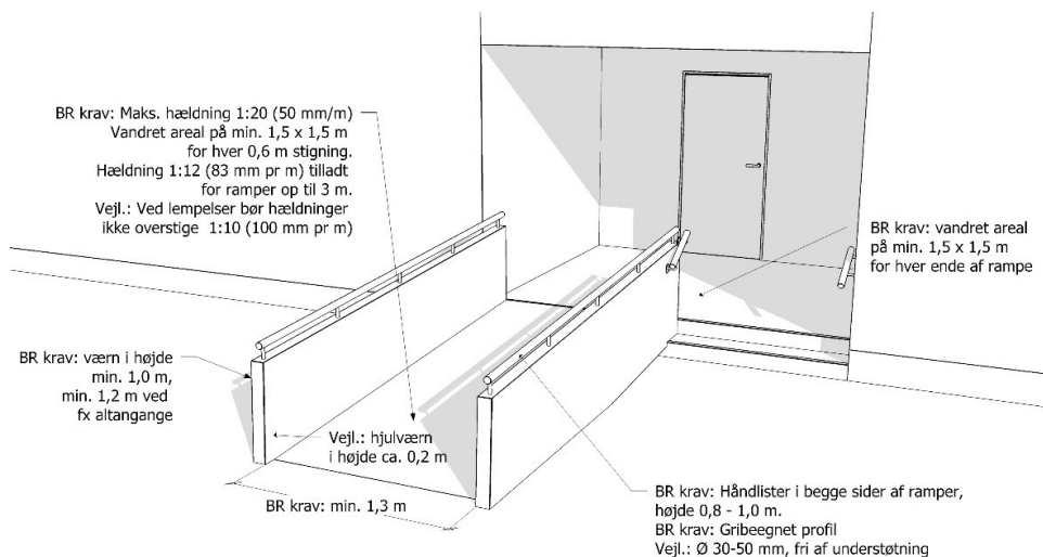
Figur 9: Eksempel på krav til rampe og supplerende trappe.
