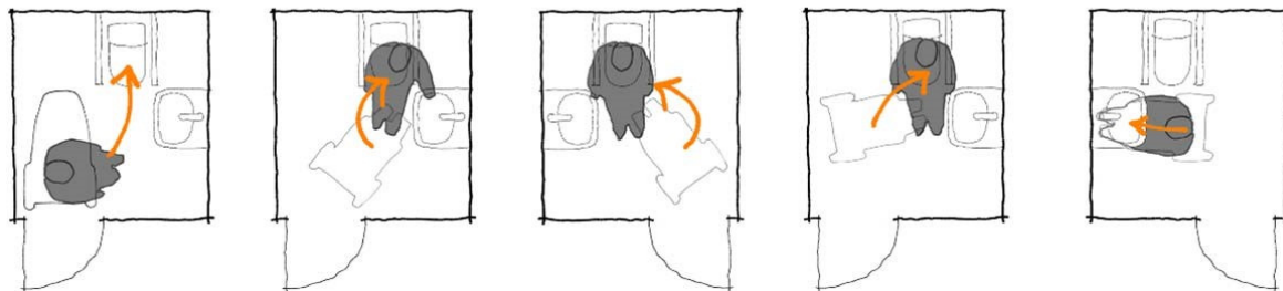
Figur 22: Vendearealet foran wc og håndvask anvendes både til manøvrering og til forflytning til wc. Pladsen på begge sider af wc'et kan også være nødvendig for en evt. hjælper. Foruden små manuelle kørestole anvender brugerne også store el-scootere og elkørestole. Behovet for hvor, stolene skal placeres, varierer stærkt efter personens funktionsnedsættelse og forflytningsmetode. Forflytning foregår oftest forfra i en vinkel til højre eller venstre. Nogle anvender kun håndvasken under toiletbesøget, fx til skift af kateter.
