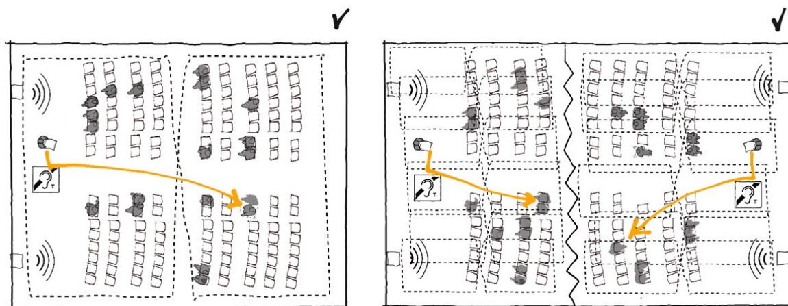
Figur 35: Store rum kan ikke dækkes af en enkelt ledningsløb langs rummets kant, da signalet bliver for ujævt fordelt. Sløjfen opdeles i flere mindre, som samlet giver en mere egnet fordeling. Et supplerende højttaleranlæg anbefales generelt, hvis alle skal kunne høre med, ligesom rummets lydregulerende egenskaber bør tilpasses dets primære formål. Der er eksempelvis forskel på de anbefalede efterklangstider for rum til tale i forhold til rum til musik. Ligger der flere rum ved siden af eller over hinanden med hver sit anlæg, bør sløjferne planlægges, så der ikke er overlap mellem de forskellige signaler. Kabler udlagt i 8-talsmønstre i modfase kan være en af metoderne. Hvis der kræves en høj grad af sikkerhed mod aflytning, kan infrarøde anlæg overvejes i stedet for teleslyngere.
