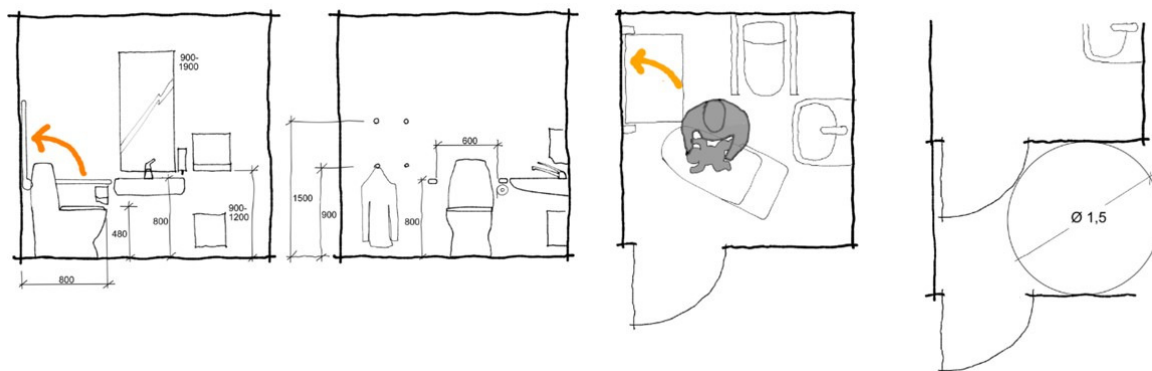
Figur 23: Eksempler på placering af udstyr i wc-rum. Bortset fra et ekstra højt wc anbringes det meste udstyr lavt af hensyn til kørestolsbrugere. Eventuelle pusleborde må ikke optage plads ved siden af wc i opklappet tilstand, og bør være mulige at klappe op med lav kraft. Vendeplads i forrum bør være fri af dørplag.
