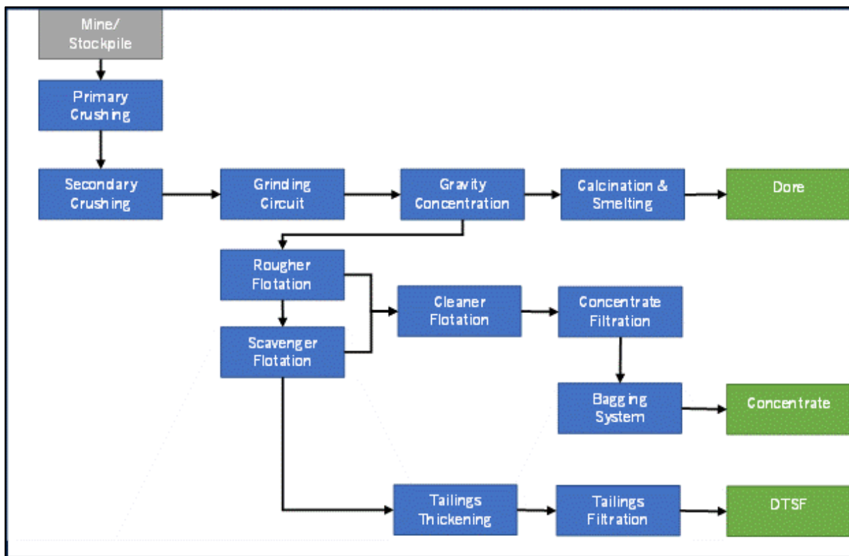
Takussutissiaq 17: Akuaanerup ingerlaneranut takussutissiaq
