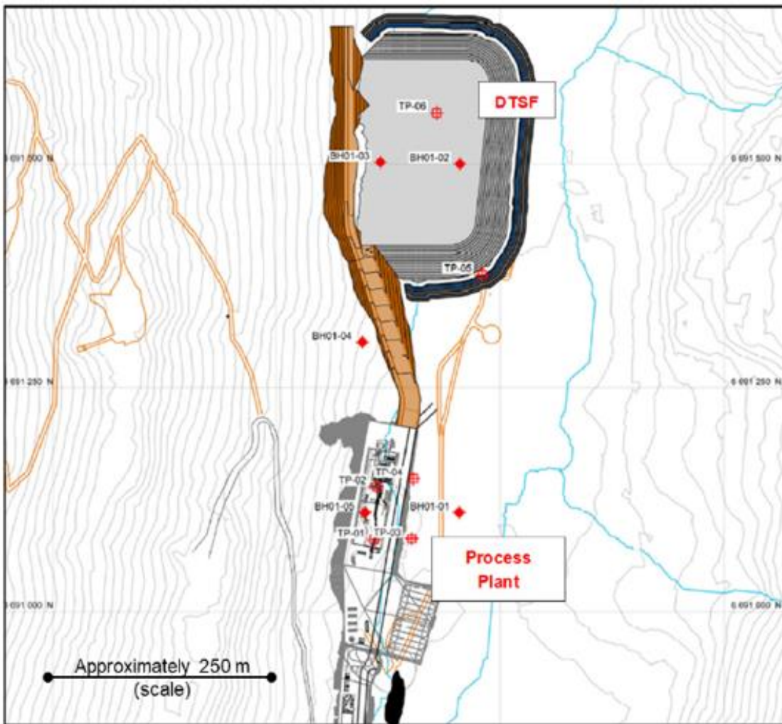
Takussutissiaq 21: Sumiiffik 3 Panertunik akuiarnerlukuusiviliorfissatut akuaaviliorfissatullu siunnersuutiqineqartut kiisalu sumiiffiit misissuiffiusut (Golder 2022a naapertorlugu nutartigaq)
