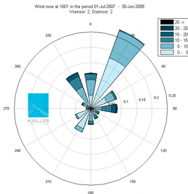
Takussutissiaq 23: Nanortalimmi 2007-imi juulimiit juni 2009-mut anoraagajuttut
