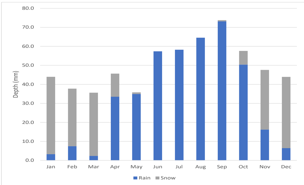
Takussutissiaq 22: Narsarsuarmi uuttortaavimmi qaammammut agguaqatigiissillugu siallersarnera / nittaatarnera (Golder 2022e).
