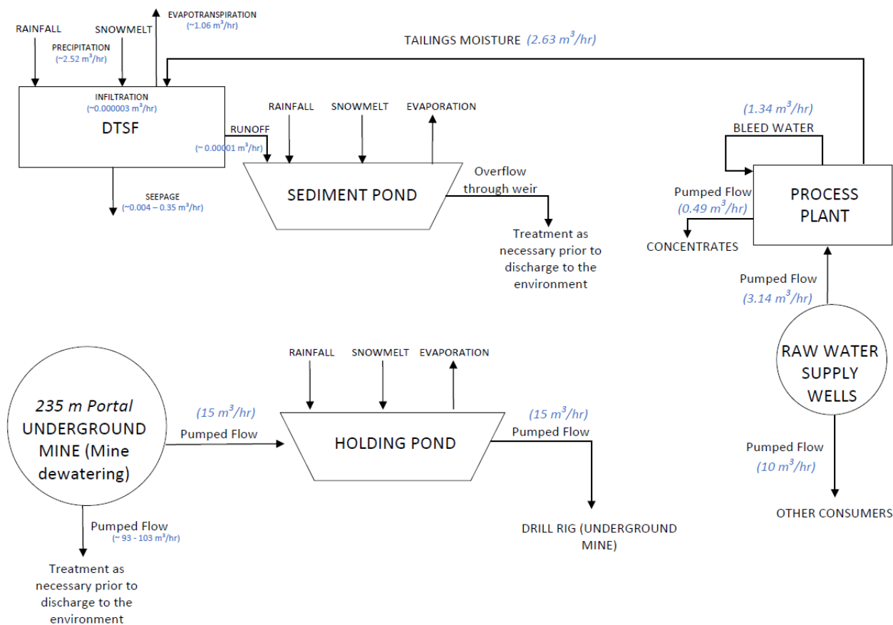
Takussutissiaq 18: Kuultisiorfimmi erngup ingerlaarnerinik takussutissiat (from Golder, 2023a)
