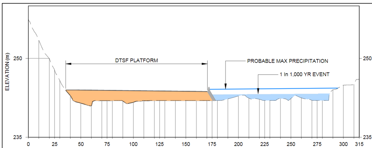
Takussutissiaq 12: Panertunik akuiarnerlukuusiviit nalinginnaasut titartagartaat, ukiuni 1000-ini ataasiarluni annerpaamik siallerujussuarneranut nittaarujussuarneranullu qarsutsivissanut sanilliullugu
