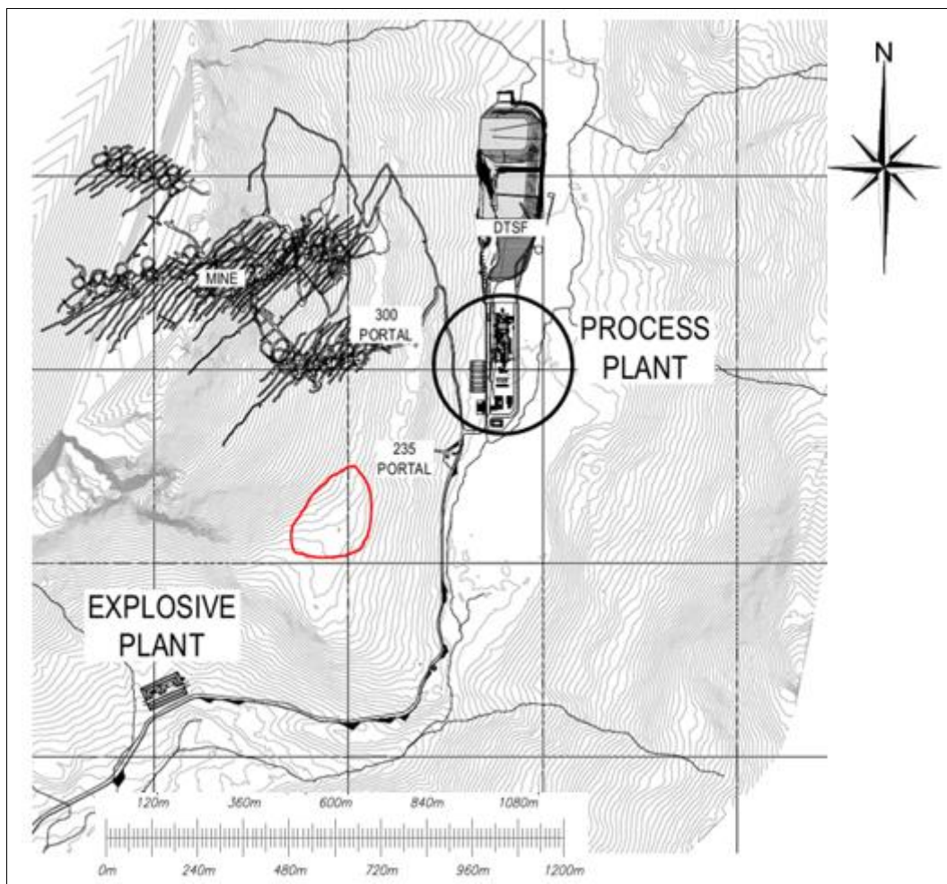
Takussutissiaq 19: Ujarakoofiussinuasumut takussutissiaq (aappalaartumik avatiligaq)
