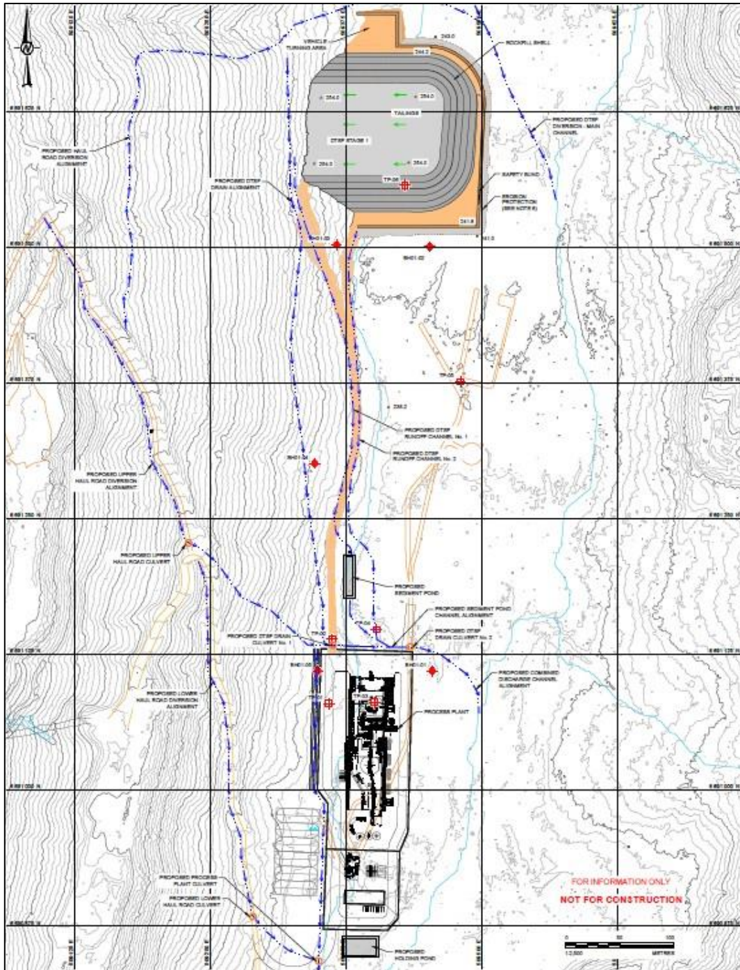
Takussutissiaq 13: Aatsitassarsiorfiup pingaarnersiorlugu titartagataa
