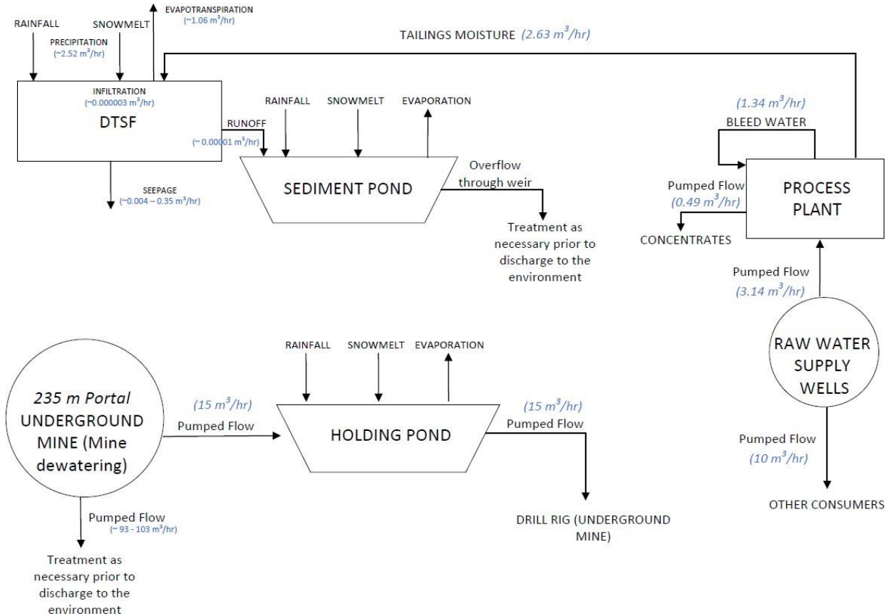
Takussutissiaq 16: Kuultisioffimmi erngup ingerlaarnerinik takussutissiat (Golder, 2023a-mit)
