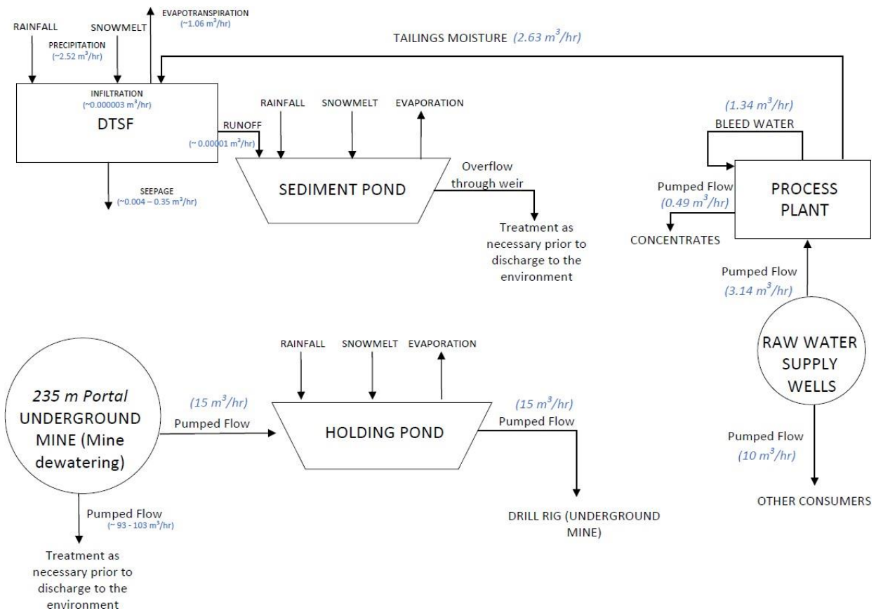
Takussutissiaq 18: Kuultisiorfimmi erngup ingerlaarnerinik takussutissiat (Golder, 2023a-mit)
