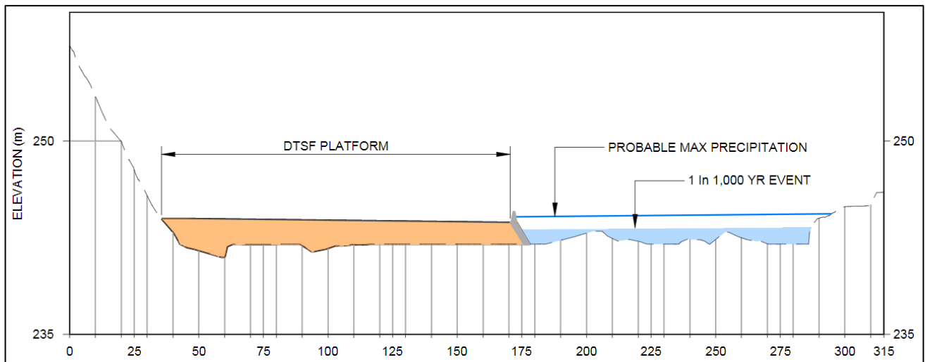
Takussutissiaq 12: Panertunik akuiarnerlukuusiviit nalinginnaasut titartagartaat, ukiuni 1000-ni ataasiarluni annerpaamik siallerujussuarneranut nittaarujussuarneranullu qarsutsivissanut sanilliullugu.
