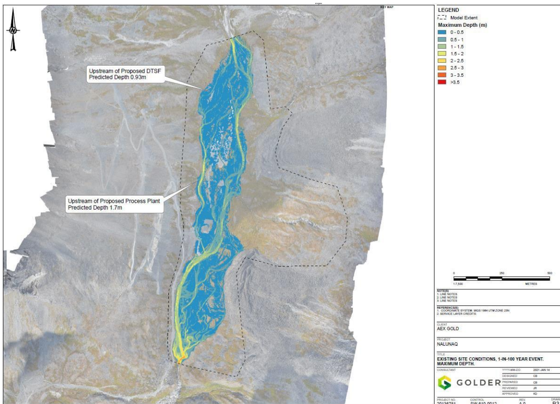
Takussutissiaq 24: Ukiut 100-t ingerlaneranni ataasiarluni qarsutserujussuarnerata itinerpaaffia ( Golder, 2022e-mit)
