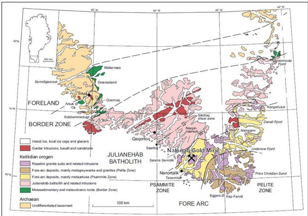
Takussutissiaq 3: Nunatta Kujataani Nunap assinga ujarassiornikkut takussutissiaq Nalunaq Mine ilanngullugu takussutissaralugu (Secher et al.-mit, 2008)
