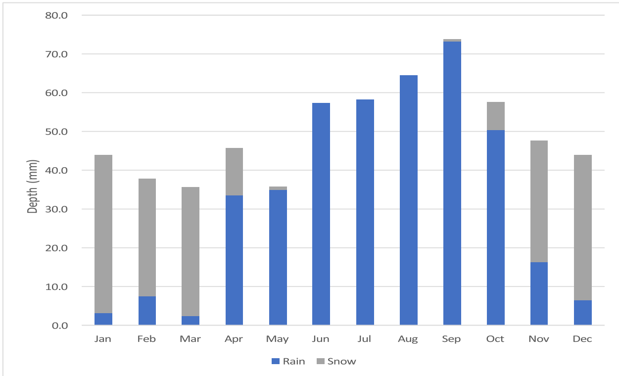
Takussutissiaq 21: Narsarsuarmi uuttortaavimmi qaammammut agguaqatigiissillugu siallersarnera / nittaatarnera (Golder 2022e).
