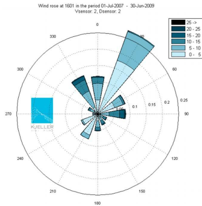
Takussutissiaq 22: Nanortalimmi 2007-imi juulimiit juuni 2009-mut anoraagajuttut
