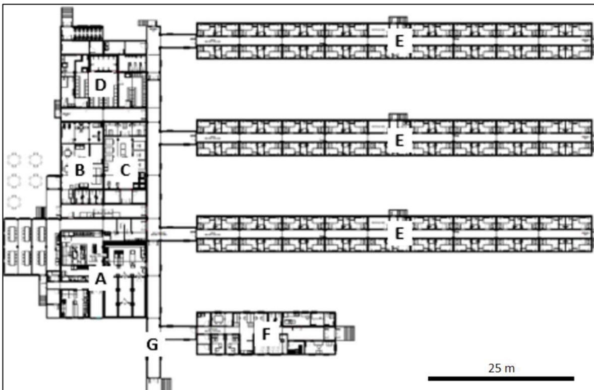
Takussutissiaq 9: Najugaqarfiup titartaqqissaarnera
