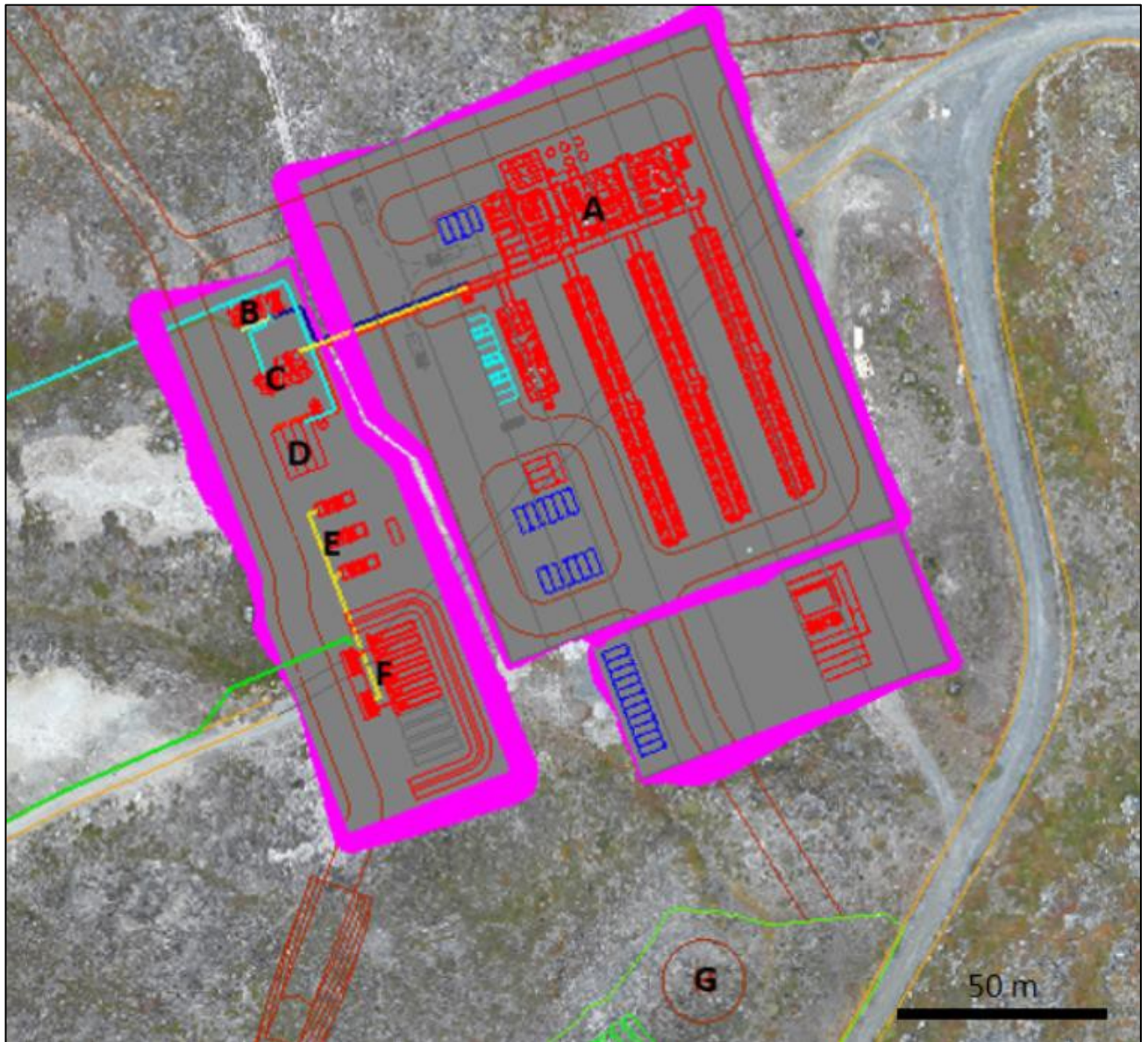
Takussutissiaq 6: Najugaqarfimmi atortulersuutit pingaernerit aaqqissorneri (A: Najugaqarfimmi atortut. B: Imermik saliivik angallattaq. C: Anartarfiit ergannik saliivik. D: Qatserutit erngat. E: Najugaqarfimmi sarfaq. F: Orsussaassivik. G: Tammaarfiup mittarfia.)
