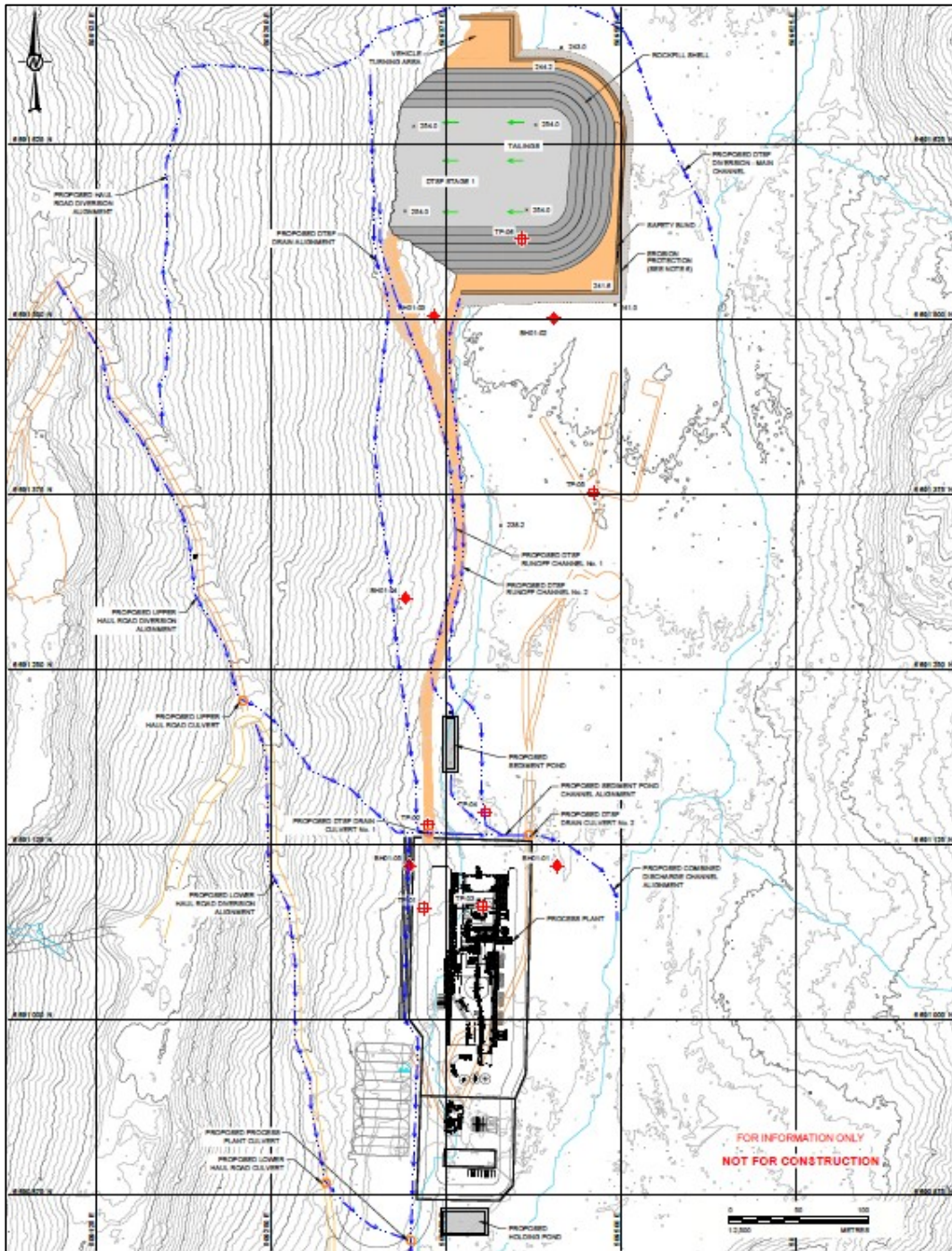
Takussutissiaq 13: Aatsitassarsiorfiup pingaarnersiorlugu titartagartaa
