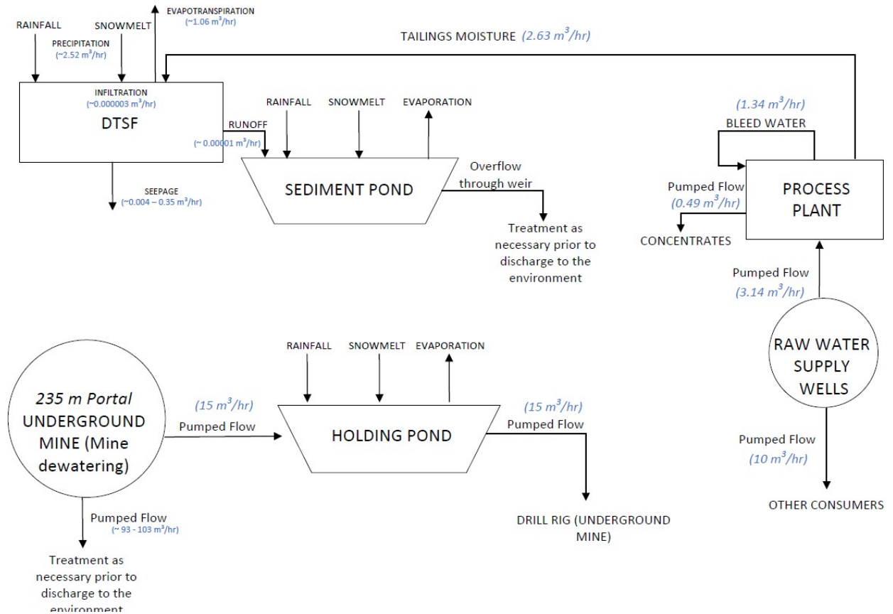
Takussutissiaq 16: Kuultisiorfimmi erngup ingerlaarnerinik takussutissiat (Golder, 2023a-mit)
