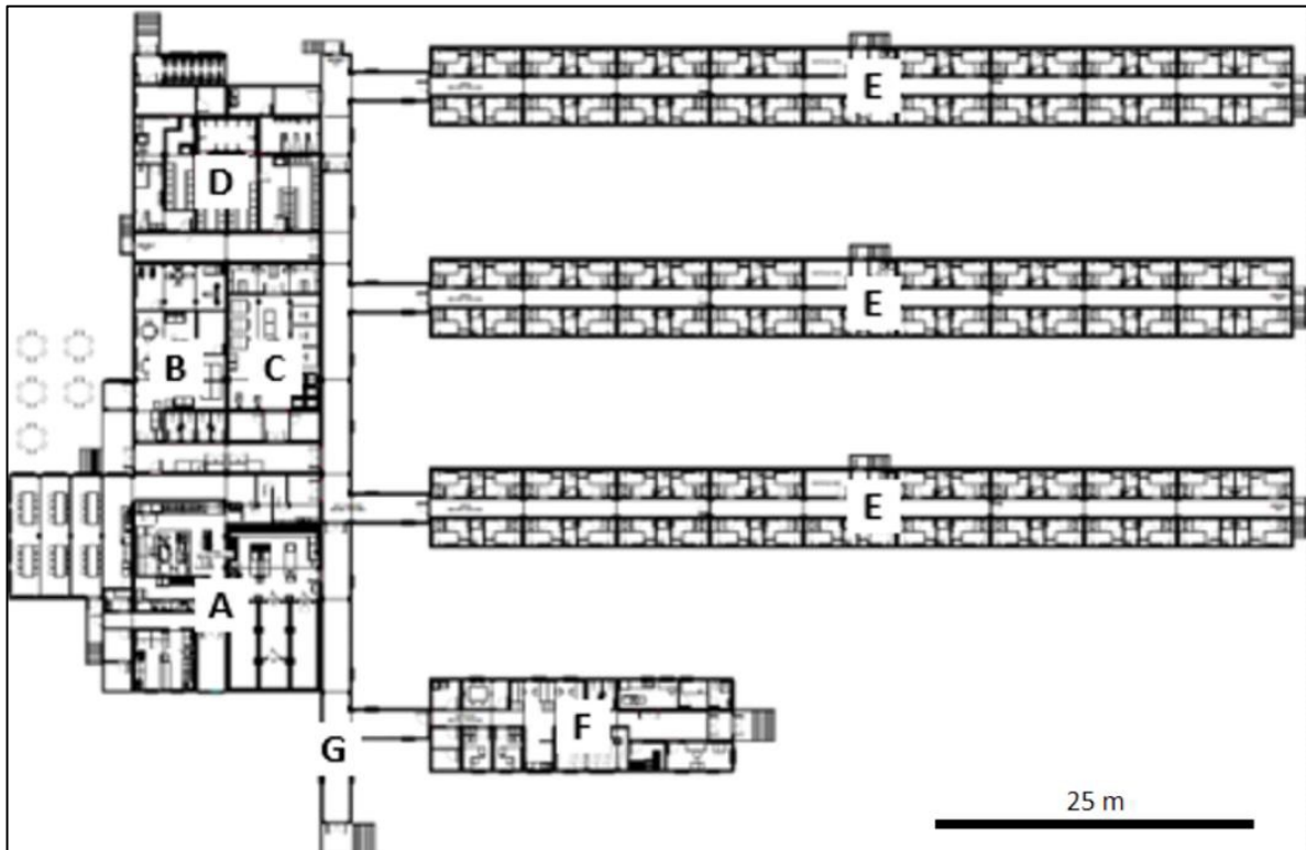
Takussutissiaq 7: Najugaqarfiup titartaqqissaarnera
