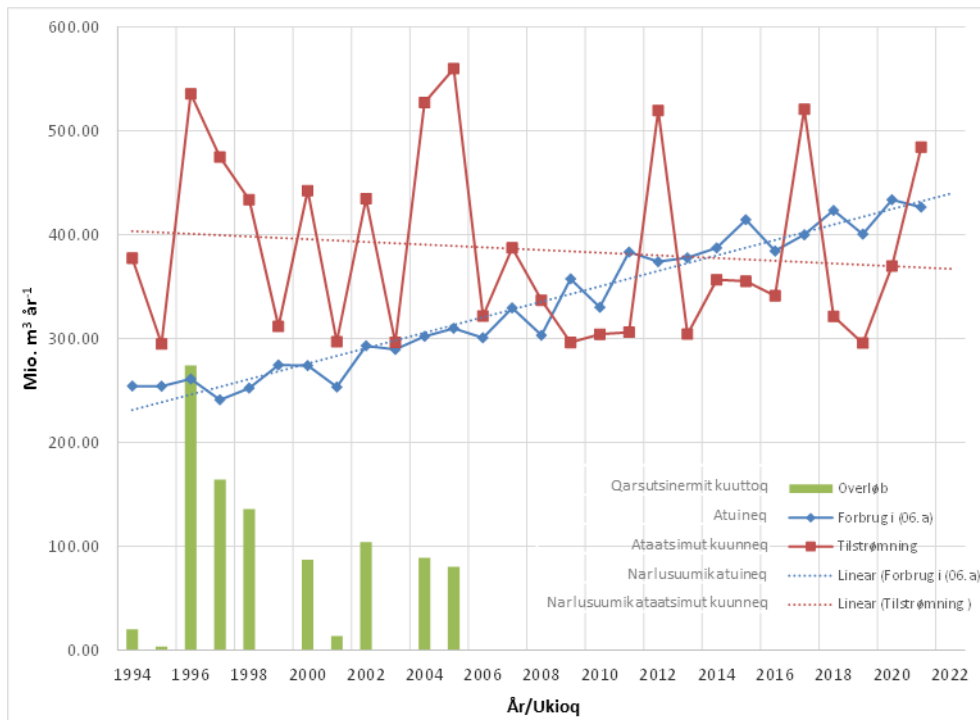
Figur 28: Ukiumoortumik engup ingerlaartarnera, utsertarnera aamma imeq nioqqutissiornermut atornerqartartoq (mio m 3 uki-umut -1 ) piffissami 1994-2021 (Nukissiorfinit paasisutissat).
