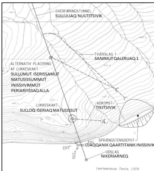
Figur 3: Sullorsuaq erngup aqqtissaa ISTA-p aamma KANG-p akornanni ((titartakkanit nr. 010-mit aamma 011-mit tigulaakkat aalajangiinissamut siunnersuummi (INUPLAN A/S, NIRAS Greenland A/S og AFRY, 2020)
