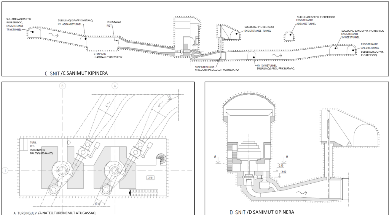
Figur 5: Innaallagissiorfik nutaaq 2 titartagartaa aamma sanianit titartagaq (titartakkap nr. 021-p ilaa aalajangiinissamut siunnersuummi) (INUPLAN A/S, NIRAS Greenland A/S og AFRY, 2020).
