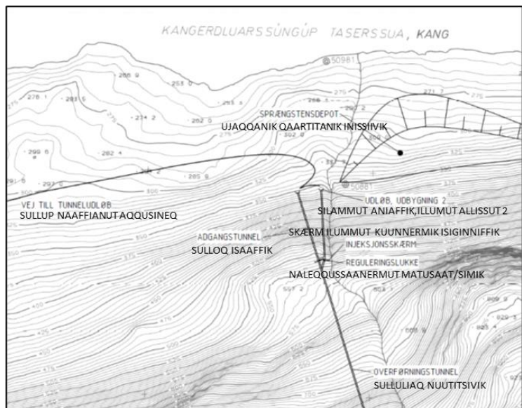
Figur 3: Sullorsuaq erngup aqqtissaa ISTA-p aamma KANG-p akornanni ((titartakkanit nr. 010-mit aamma 011-mit tigulaakkat aalajangiinissamut siunnersuummi (INUPLAN A/S, NIRAS Greenland A/S og AFRY, 2020)
