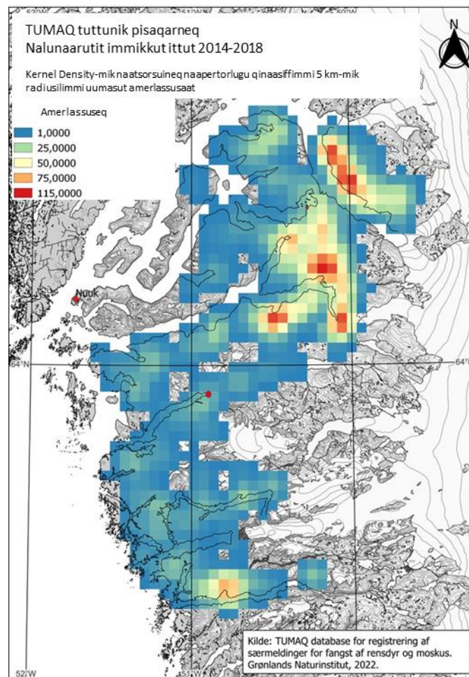
Figur 36: Ameralimmi tuttoqarfimmi aavarluni pisaqartarnek piffissami 2014-2018. Ameralimmi aamma Nuup Kangerluani pisaqartoqarnerusarpoq, kisianni aammattaaq Utoqqarmiut Kangerluarsunnguanni aamma KANG-mi pisaqartoqartarpoq. Toorneq appalaartoq Utoqqarmiut Kangerluarsunnguata qingvaniittoq taassaavoq imermit nukissiorfik.
