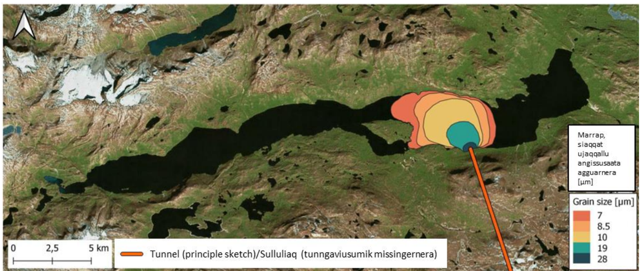
Figur 33: Pisuusaartitsilluni naatsorsuinerit takutipaat kuuttut naqqanut kinnerat ISTA-meersut KANG-mit kuunnermit kingornatigut (Niras, 2022a).
