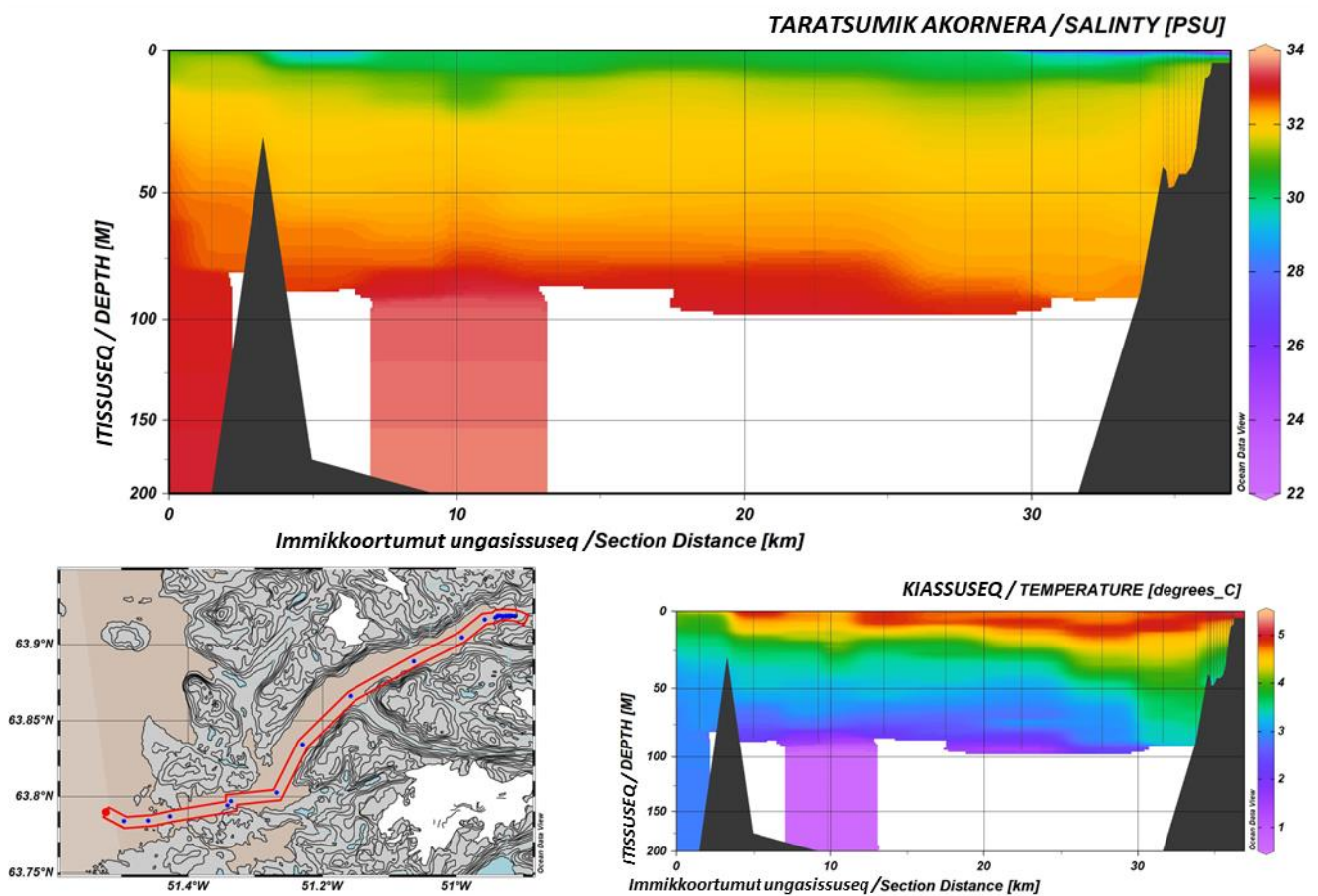
Figur 31: Utoqqarmiut Kangerluarsunnguani. Tarajoqassuseq aamma kiassuseq/nillissuseq nunap assiliaralugu CTD-mik kangerluk sinerlugu uuttortaaneq tunngavigalugu septembari 2021. Ilutsini matoqqasuni qinertuni takutinneqarpoq naqqata nalingajaaniittut sumiiffinni ittissutit tunngavigalugu, uani taamaallaat takuneqarsinnaapput kangerlummi ikkannerniittut erngup tarajoqanngitsup aniaffiata eqqaani. Takuneqarsinnaasut annersaannut ilaapput immap qaava 80-100 m. Itinersat takusutissiami ilanngunneqarput itinersani inernerit takutinniarlugit 200 m. kitaani (ungasissuseq 0 km.) aamma kangiani (ungasissuseq 10 km. aallaaviani (malugiuk ittissuseq siaarneqarmat sivingassutit qaavaniittut erseqqinnerulersinniallugit). Erseqqissumik takuneqarsinnaapput immap qanoq issusiata assigiinnigissutaa ittissutimi >100 m. killiffiup iluani aamma avataani. Kisisitit takutippaat sumiiffimmi imaq akuleriittoq itinermi pulasut aamma ukiuunerani immap ingerlaarnera. Malugiuk imeq tarajoqanngitsog aamma kiassutsip/nillissutsip qaavani
