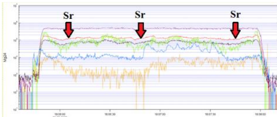
Figur 23: KANG: Misissuinerit inernerinut assersuut eqaluk 56 cm. tatsimi KANG-mi – Strontium-ip akulerussimanerata allanngornera soqutaavallaangilaq (Sr-ip kimittussusia) sissik qupillugu, tassa imaappoq aalisakkap imaaniissimanera malunnangilaq
