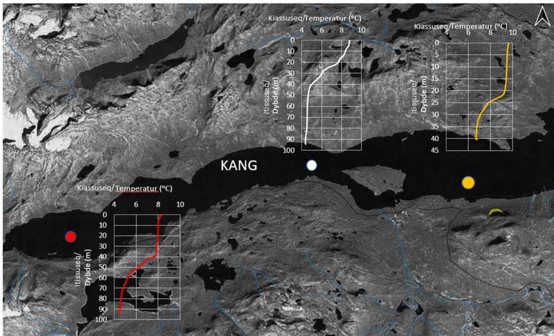
Figur 9: CTD-mik uuttuut atorlugu KANG-mi septembarimi 2021-mi uuttortaanernut takussutissiaq.
