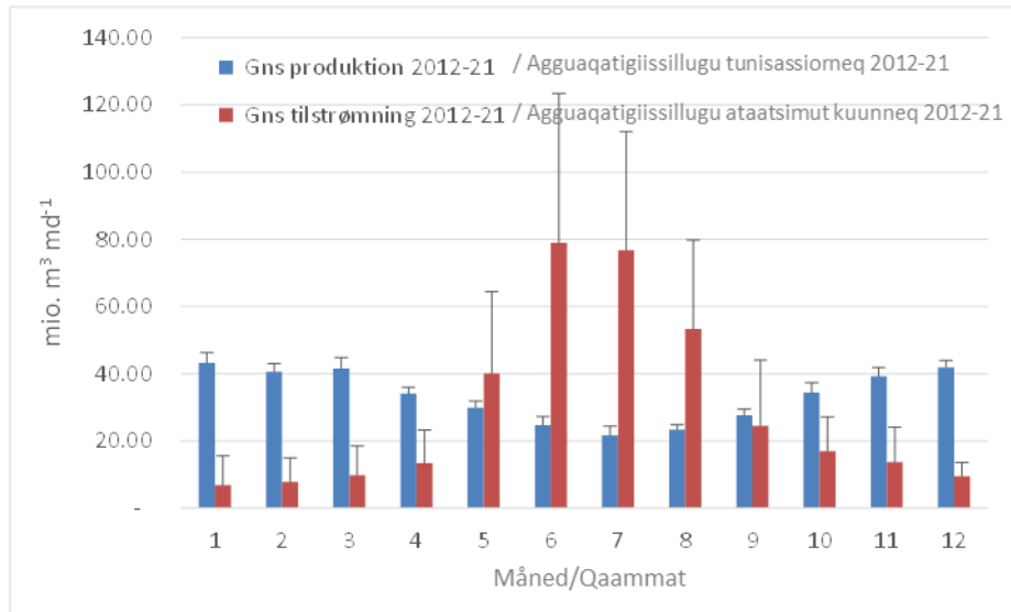
Figur 29: Piffissap ingerlanerani erngup KANG-mut kuuttarnera (ilimanarnerusoq) taamatullu aamma imeq nioqutissiornermut atorineqartartoq (mio m 3 md -1 ) siuertamut (+nalinginnaasumik nikerarneq) ukiut qulit ingerlanerini 2012-mit 2021-mut (Nukissiorfinnit paasisutissat).
