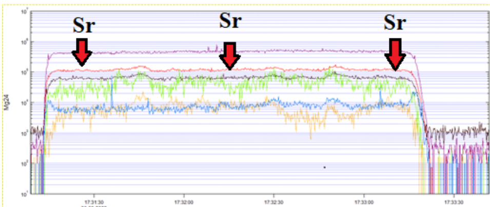
Figur 24: ISTA: Misissuinerit inernerinut assersuut eqaluk 33 cm. tatsimi ISTA-mi – Strontium-ip akulerussimanerata allanngornera soqutaavallaangilaq (Sr-ip kimittussusia) sissik qupillugu, tassa imaappoq aalisakkap imaaniissimanera malunnangilaq.
