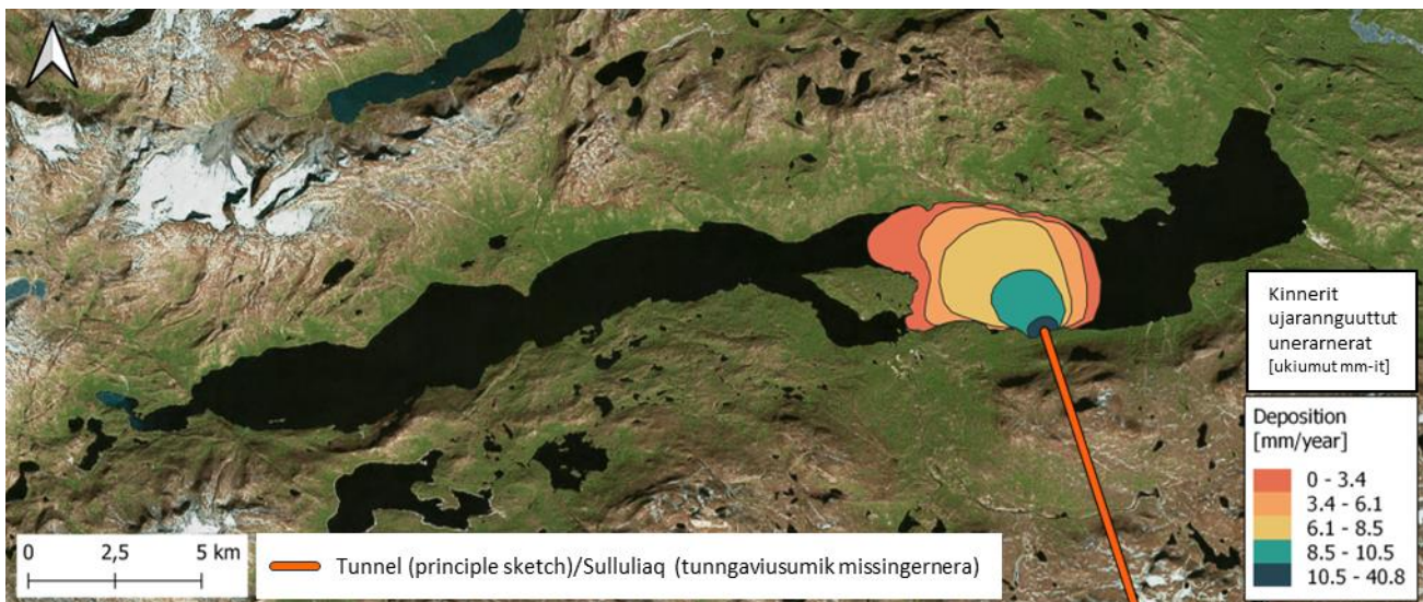
Figur 26: Tatsimut kinnerit (mm) ISTA-mit KANG-mut erngup kuuffiani aamma eqqaani.
