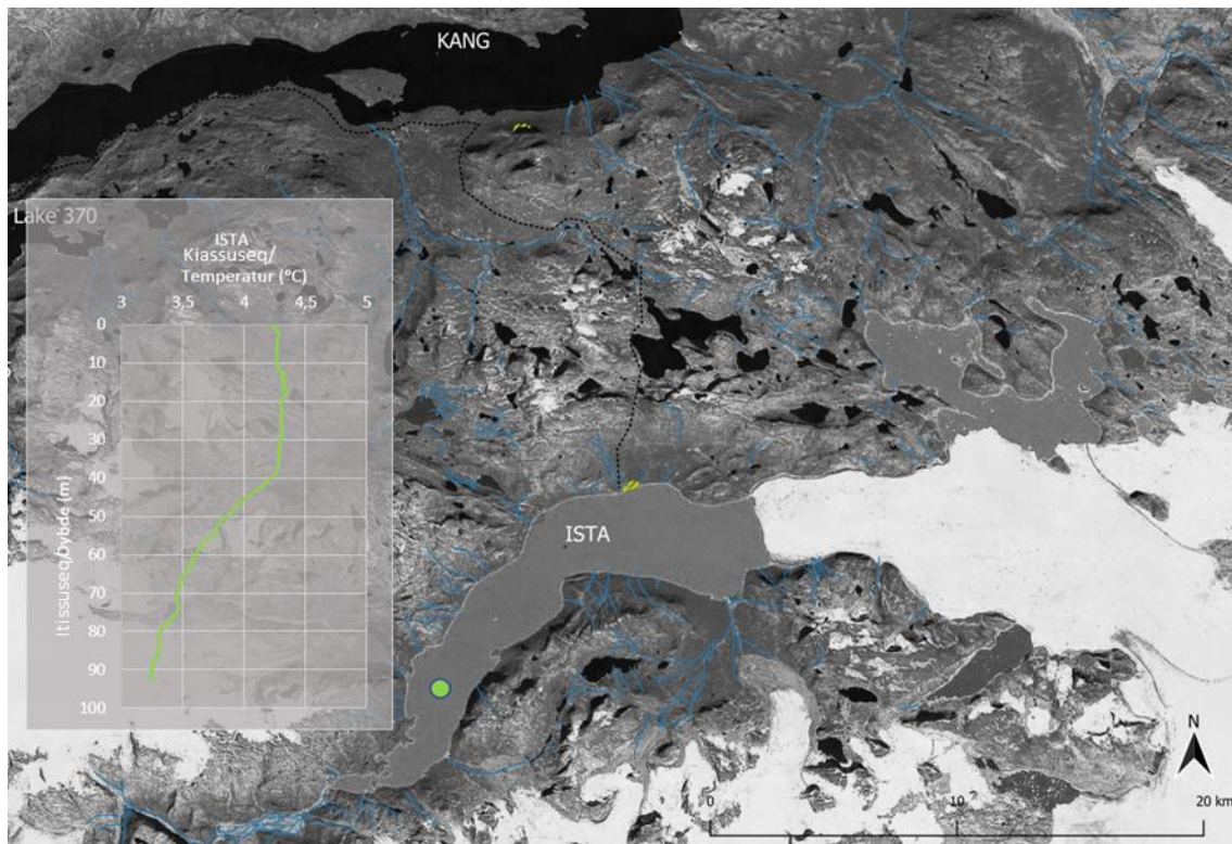
Figur 11: CTD ilisarnaataa ISAT-mit septembari 2021.
