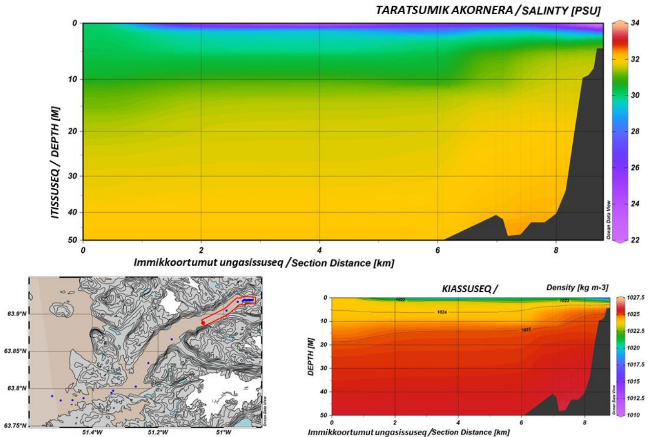
Figur 32: Utoqqarmiut Kangerluarsunnguata qinnguani immammi ikerinnarmi 50 meterisut ittussilik misissorneqarpoq. Tarajoqasusia aamma ussissusia tassani tunngavineqarput CTD-mik uuttortaanerit septembarimi 2021 (paasissutissat matuma siulianiittut assingi). Paasissutissami erseqqissarneqarpoq erngup tarajoqanngitsup akulerukkiartorneq kangerlummi avammukariartornermini (malugiuk ittussisip uuttornera ammuksartoq allisinneqarpoq). Usissutsimi takutinneqarpoq akulerussimasut 10 meterinik ittussilimmi, tamannalu taamaappoq kangerluk tamakkerlugu kangerluup paavani immap qaavani akulerussineq suli ingerlavoq.
