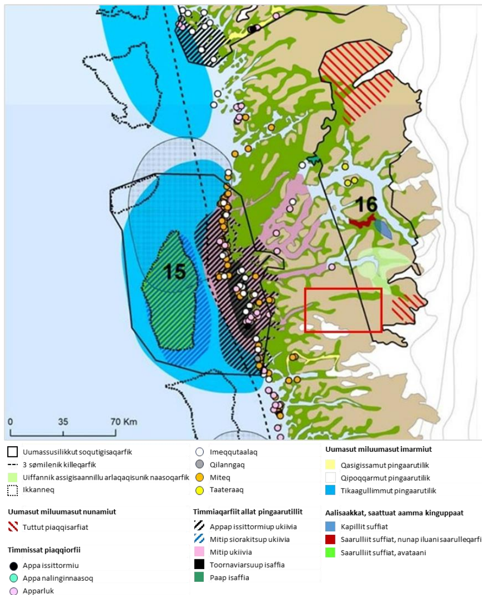
Figur 34: Suliniutip sumiiffiani uumassusillit sumiiffii soqutiginarlut Utoqqarmiut Kangerluarsunnguanni innaallagissiorfiup allineqarnerani. Suliarinnittut Christensen et al. (2016). Suliniutip sumiiffia kipparissup aappalaartup iluaniippoq. Naasut assigiinngiaartut KANG-p avannamut kimmur amerlisimapput qorsummik qaamasumik sumiiffimmi 16-imi ilisarnaaserneqarsimapput.
