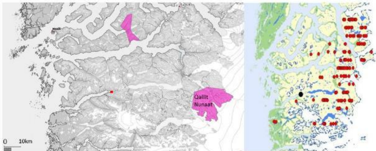
Figur 37: Saamerleq, tuttu piaqqiortarfiat Qallit Nunaat Utoqqarmiu Kangerluarsunnguanni imermit nukissiorfiup kangiani (kipparisoq aappalaartoq) (Grønlands Selvstyre , 2022). Talerpilleq, tuttu takuneqarfiat (ammalortoq aappaluttoq) Ameralimmi uumasogatigiinnik kisitsisoqarnerani 2021, Utoqqarmiu Kangerluarsunnguanni imermit nukissiorfik qernertumik ammalortumik nalunaarneqarpoq, suliarinnittunit (Cuyler, Nymand, Jensen, & Mølgaard, 2016)
