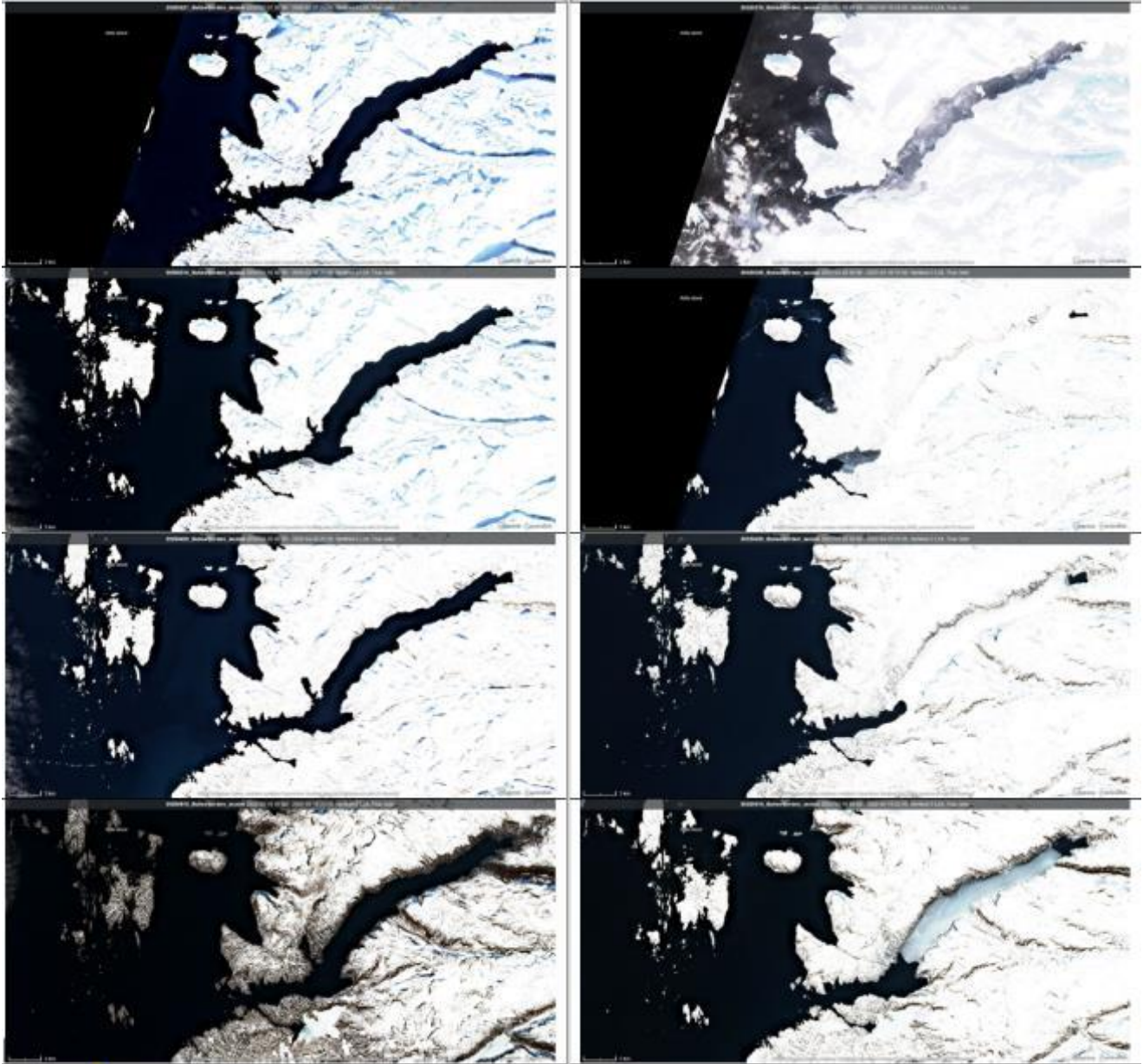
Figur 30: Satellit-imit assilisat, taakkunani takutinneqarpoq Utoqqarmiut Kangerluarsunnguanni ukiuunerani sikuunera 2020 (saamerleq) aamma 2022-mi (talerperleq) piffissaq ingerlasoq qaammatikkaarpoq februaarimit (qulleq) maajimut (alleg). Malugiuk sumiiffik sikoqanngitsoq 2022-mi kangerluup qinnguani tassaniippoq sullorsuarmit erngup kuuffia. Tigusiffik: https://apps.sentinel-hub.com/eo-browser .
