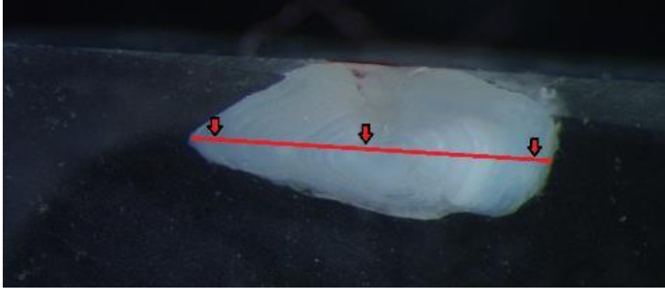
Figur 22: Sissik titarneq tassaavoq laseri, sissik ilaatigut Strontium-imik (Sr) akoqarnersoq misissorniartuq, paasinia-reqarpoq aalisagaq imaaniissimanersoq.
