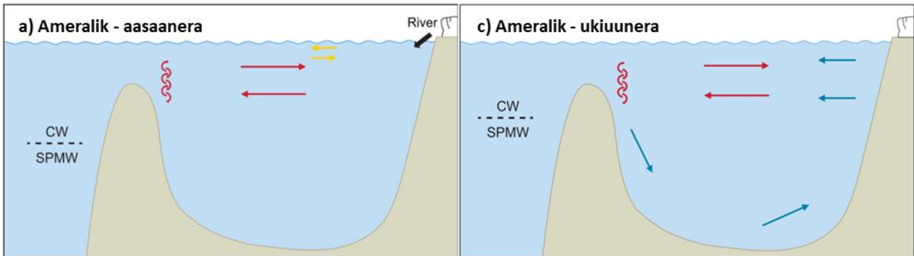
Figur 27: Titartaganngorlugu takussutissiaq kaaviiaartut isikkui pingaarnertit assaanerani aamma ukiuunerani Utoqqarmiut Kangerluarsunnguata eqqaaniittumi kangerlummi Ameralimmi, taanna aammattaq imermik tatsineersunik akuneqartarpoq aamma imatut itivallaartorsuunani 110 m. Qarsuusat silittut qernertut takutippaat imeq tarajoqanngitsoq kuutsigut imaanut kuuttoq. Qarsuusat amitsut takutippaat 1) estuarin cirkulation (sungaartut), 2) baroklin cirkulation ikerinnarmi (aappalaartoq) kiisalu 3) itisuumi immap sinerissameersup akulerunnera (tungujortoq) (assilineqarpoq uannga (Stuart-Lee, Mortensen, Kaaden, & Meire, 2021).
