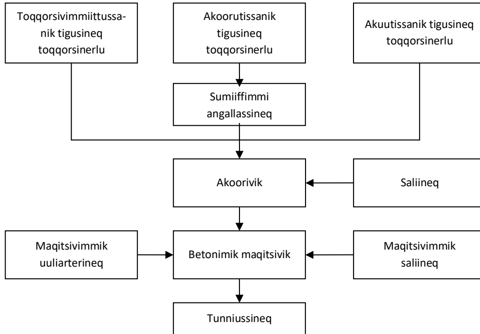
Takussutissaq 1: Betoniliornermi ingerlanissaanut diagrammi (uangaanneersoq: Branchebilag for B 202 – tak. imm. 15).
