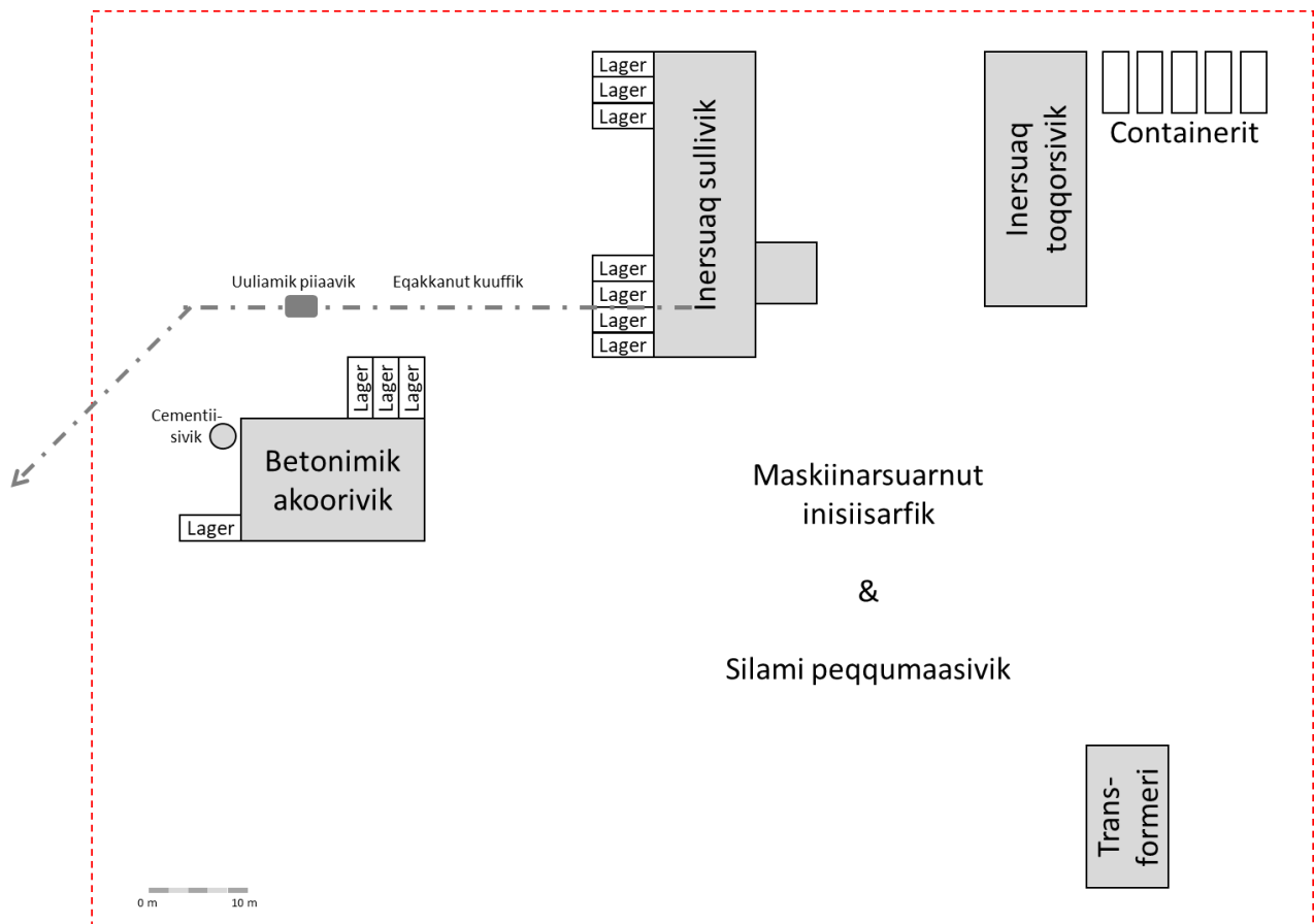
Takussutissaq 1 Nunaminertamut betoniliorfimmik inissiiviusumut maskiinanut atortunullu il.il. inissiivittalimmut assersuut
