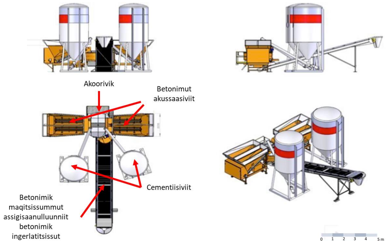
Takussutissaq 2 Betoniliorfiup nuunneqarsinnaasup ilusaanut assersuut (Fibo Intercon)
