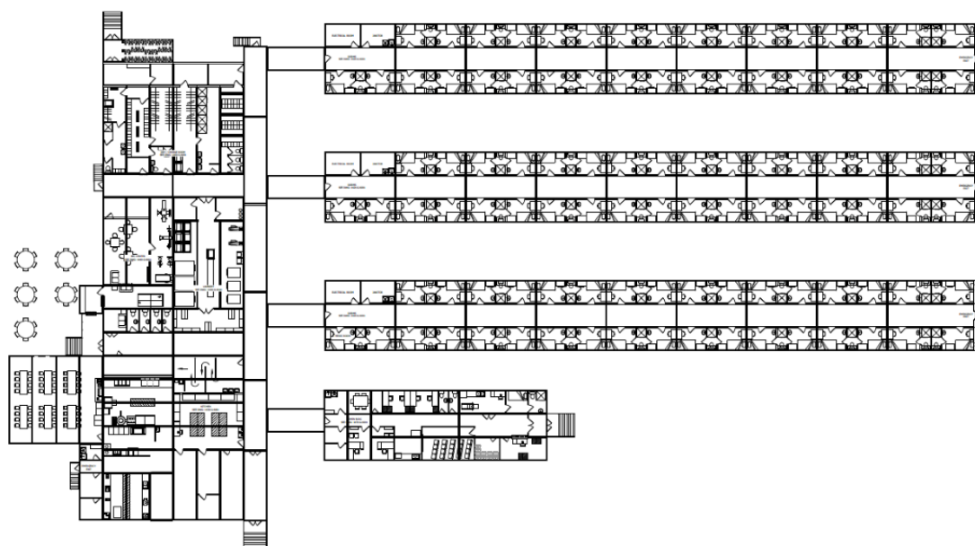
Figur 3: Forslag til indretningen af lejren og lejrkomplekset.
