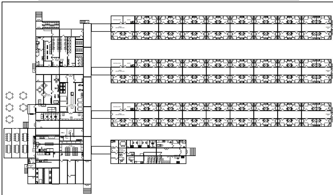
Takussutissiaq 3: Tammaarfimmi sanaartukkat aamma najugaqarfissap isikkussaatur siunnersuutigineqartoq
