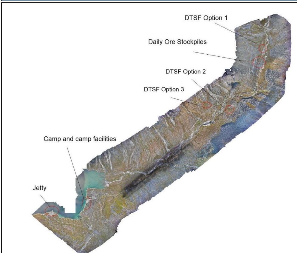
Takussutissiaq 1: Nalunaq Gold-imik suliniuteqafik suliniutip ilaannut pingaarnernut sumiiffiit siunnersuutigineqarsimasut ilanngullugit. Nunap assingi annikitsortaanik aamma ilanngussisut suliniutip allaaserineqarnerani ataani nassaarineqarsinnaapput.
