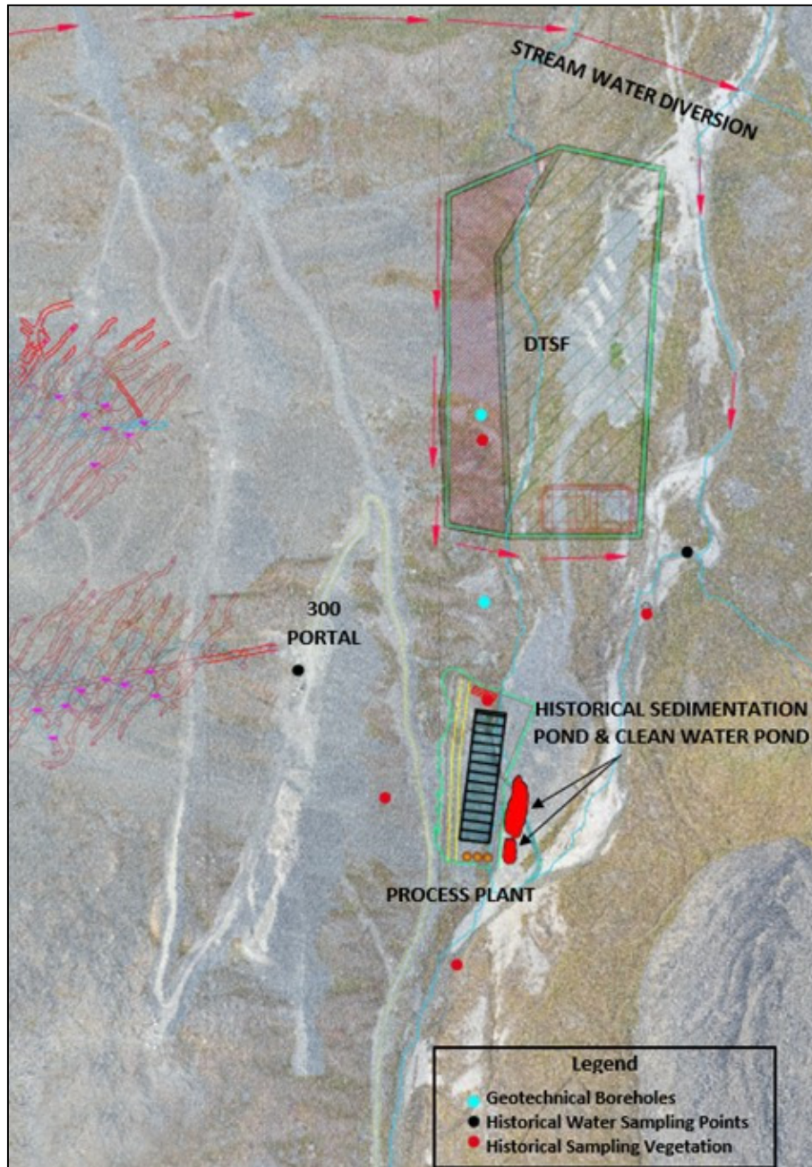
Takussutissiaq 11: Aatsitassarsiornermi sinnikunut panertunut qaleriissaaraluni toqqorsiviup (DTSF) inissaatut siunnersuutigineqartoq.
