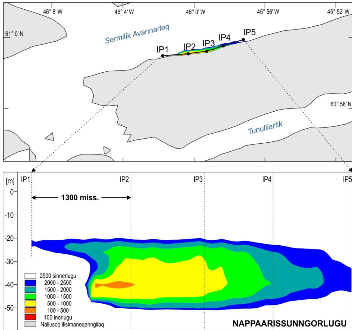
Ilusiliaq 65 Aasaanerani kuutsinneqartunut -40 m–it itissuseritillugit kimikillitsinissamut tunngavigisanut ammuinnartunut 50 procentinut inissiineq ([16] - Ilusiliaq 7-2e,f)
