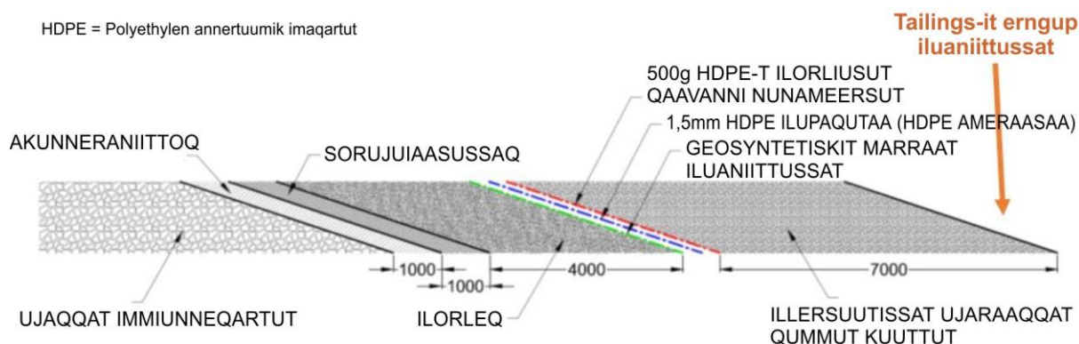
Ilusiliaq 49 Sapusiaq – Iloqutaani killormut kuuttut ([1] - Titartagaq 002-1020)
