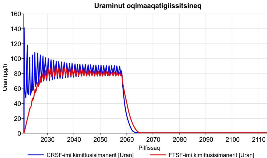
Ilusiliaq 60 FTSF-imi aamma CRSF-imi suliassap ingerlanneqarnerata nalaani uraninik kimittusisimanerit, GoldSim atorlugu naatsorsorneqartut
