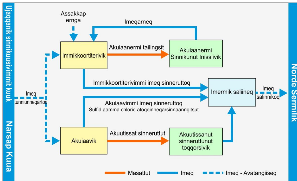
Ilusiliaq 23 Erngup oqimaaqatigiinnera
