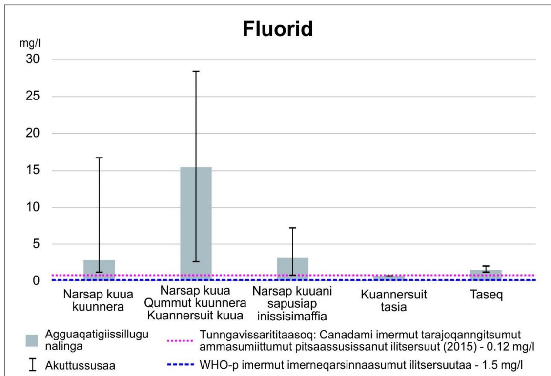
Ilusiliaq 56 Kussiorneqartumi fluoridit katersuussimanerat ([53] - Ilusiliaq 4.8)
