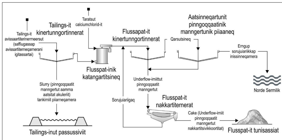
Ilusiliaq 21 Akuaavimmi imermik saliinerup ingerlaarfiinut titartaganngorlugu takussutissiaq
