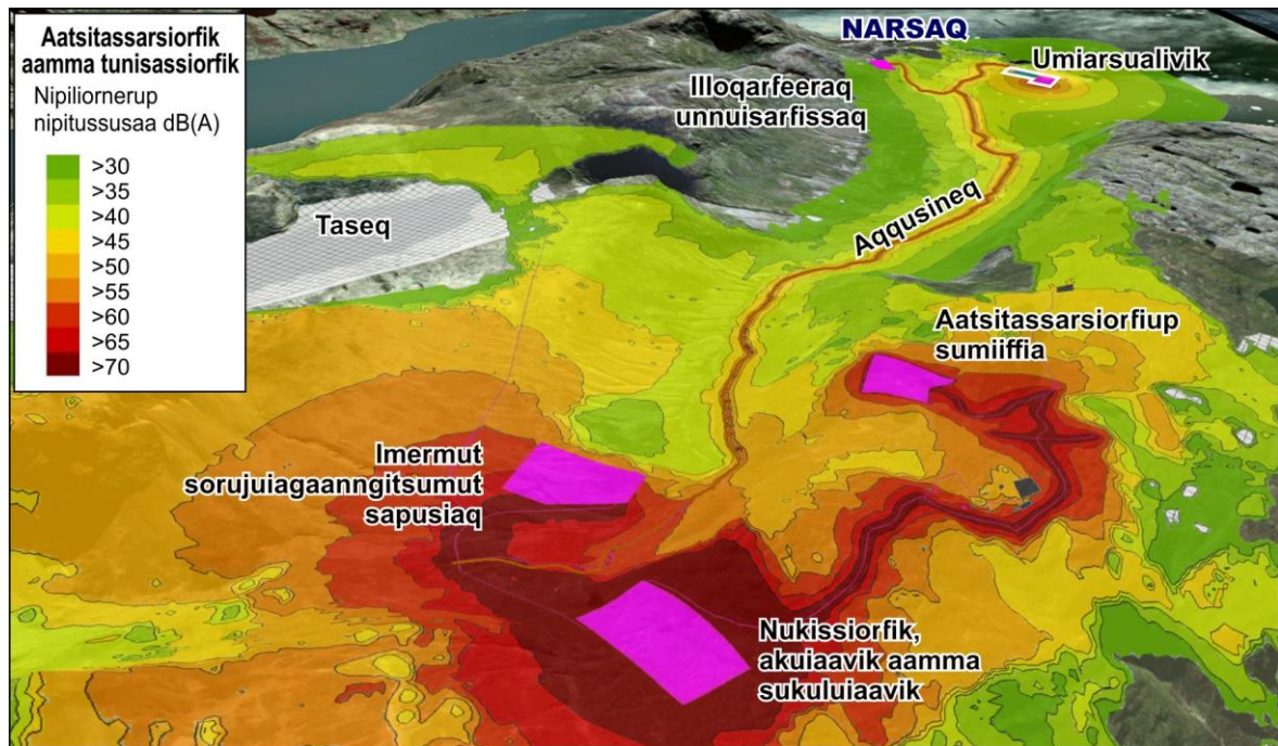
Ilusiliaq 40 Ingerlatsinerup nalaani aatsitassarsiorfimmi suliareqqiisarfirmmilu nipiliortitsinerit naatsorsorneqartut
