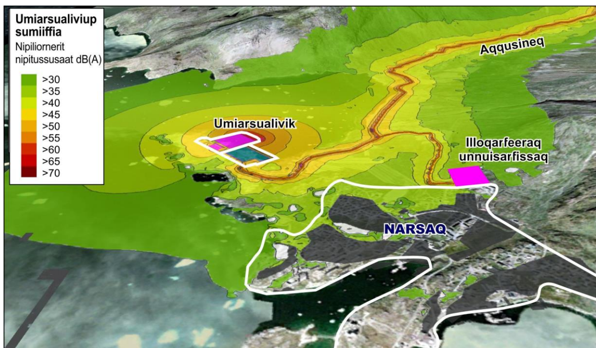
Ilusiliaq 42 Ingerlatsinerup immikkoortuani umiarsualivimmi nutaami eqqaanilu nipiliortitsinerit naatsorsorneqartut
