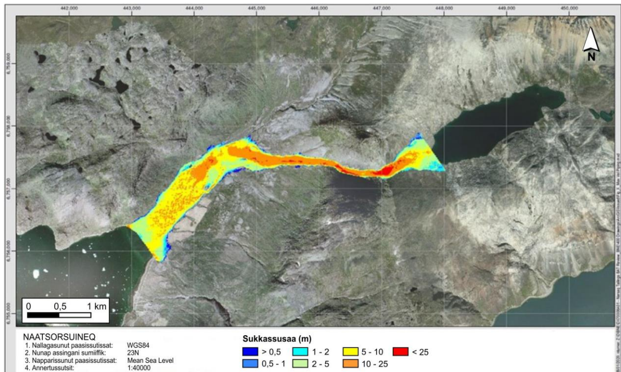
Ilusiliaq 52 Sukkassutsit annerpaaffissaat – aserortunut Rico et al.-imi (2008) aamma Froehlichimi (2008) nassuiarneqartut tunngavigalugit ([110] - Ilusiliaq 3.8)
