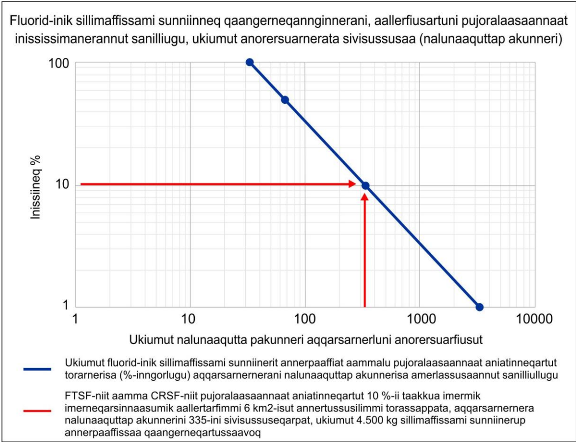
Ilusiliaq 62 10 %-inik inissiinerimi aqqarsarnerluni pisoqarnerani fluoridinik aniasoqarnerata sivisussusaa ([59] - Ilusiliaq 7-6)
