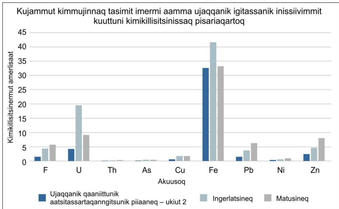
Ilusiliaq 66 Nunamiittut annertussusii imaluunniit PNEC-ni naliusut naammassiniarlugit akuusunut kimikillitsinissamut piumasaqaatit ([31] - Ilusiliaq 17)
