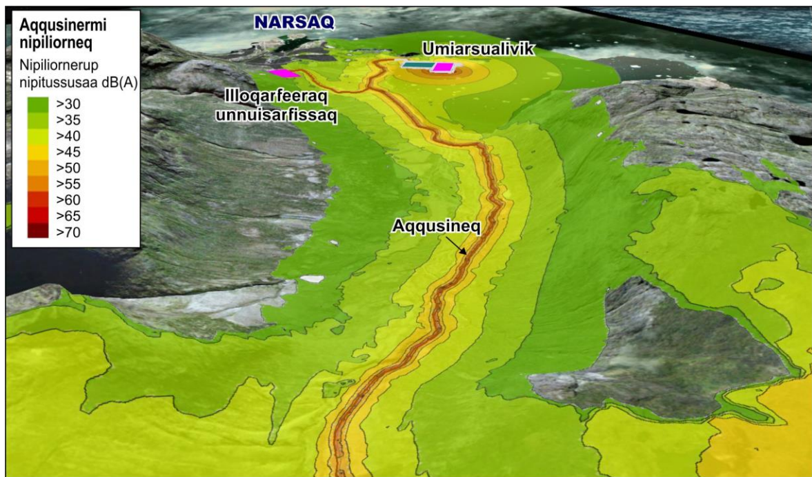
Ilusiliaq 41 Umiarsualivimmiit aatsitassarsiorfimmuut aammalu umiarsualiviup nutaap eqqaani akkusineq atuataarlugu nipiliortitsinerit naatsorsorneqartut
