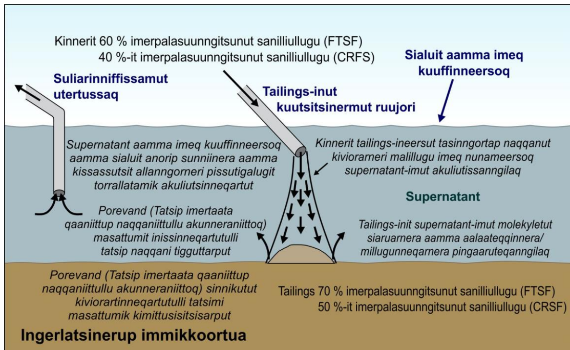
Ilusiliaq 17 Ingerlatsinerup immikkoortuanut takussutissiaq immersuganngorlugu
