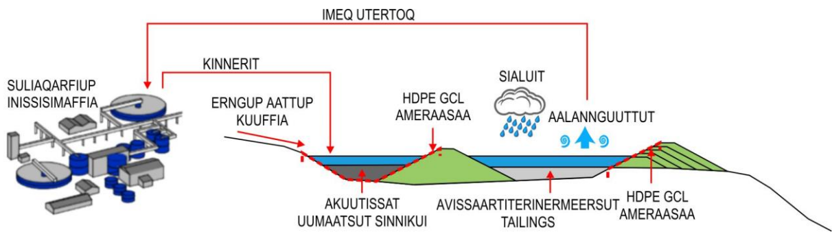
Ilusiliaq 33 Tailingsinik masattumi inissiivissap ilusiligaanera
