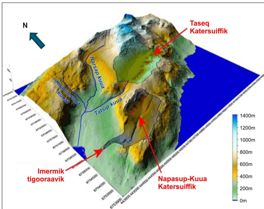
Ilusiliaq 54 Tatsip kuua aamma sumiiffiit kussiorneqartussat
