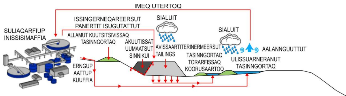
Ilusiliaq 32 Tailingsinik panertumi inissiivissap ilusiligaanera
