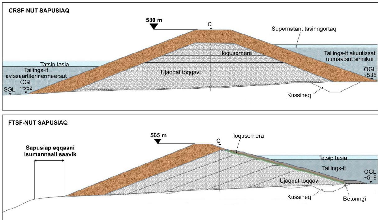
Ilusiliaq 16 tailingsinut akuutissat uumaatsut sinnikuinik akulinnut inissiisarfimmut (CRSF) (qulleq) aammalu ukiuni 37-ini tailingsinik inissiivissamut (FTSF) (alleq) sapusiap kippaata assilineria
