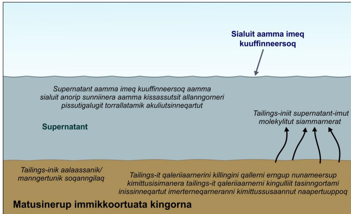
Ilusiliaq 20 Matusinerup kingorna immikkoortuanut immersuganngorlugu takussutissiaq
