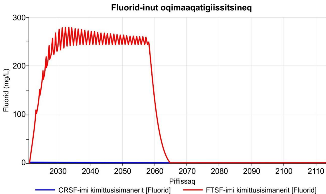
Ilusiliaq 61 FTSF-imi aamma CRSF-imi suliassap ingerlanneqarnerata nalaani fluoridinik kimittusisimanerit, GoldSim atorlugu naatsorsorneqartut
