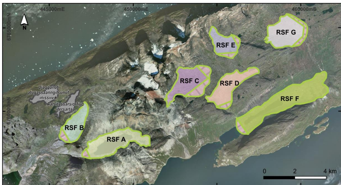
Ilusiliaq 31 Tailingsinut inissiivissamut periarfissat
