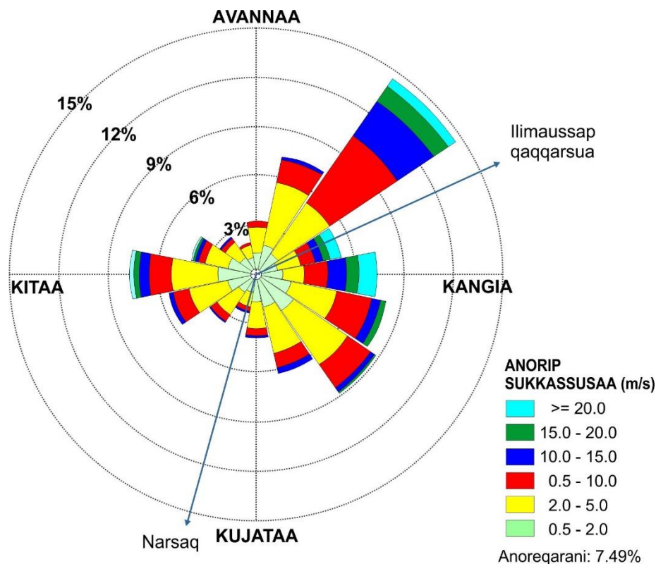
Ilusiliaq 35 Anorip sammivii aamma anorip sakkortussusii Kuannersuarni silasiorfimmi nalunaarsorneqartut
