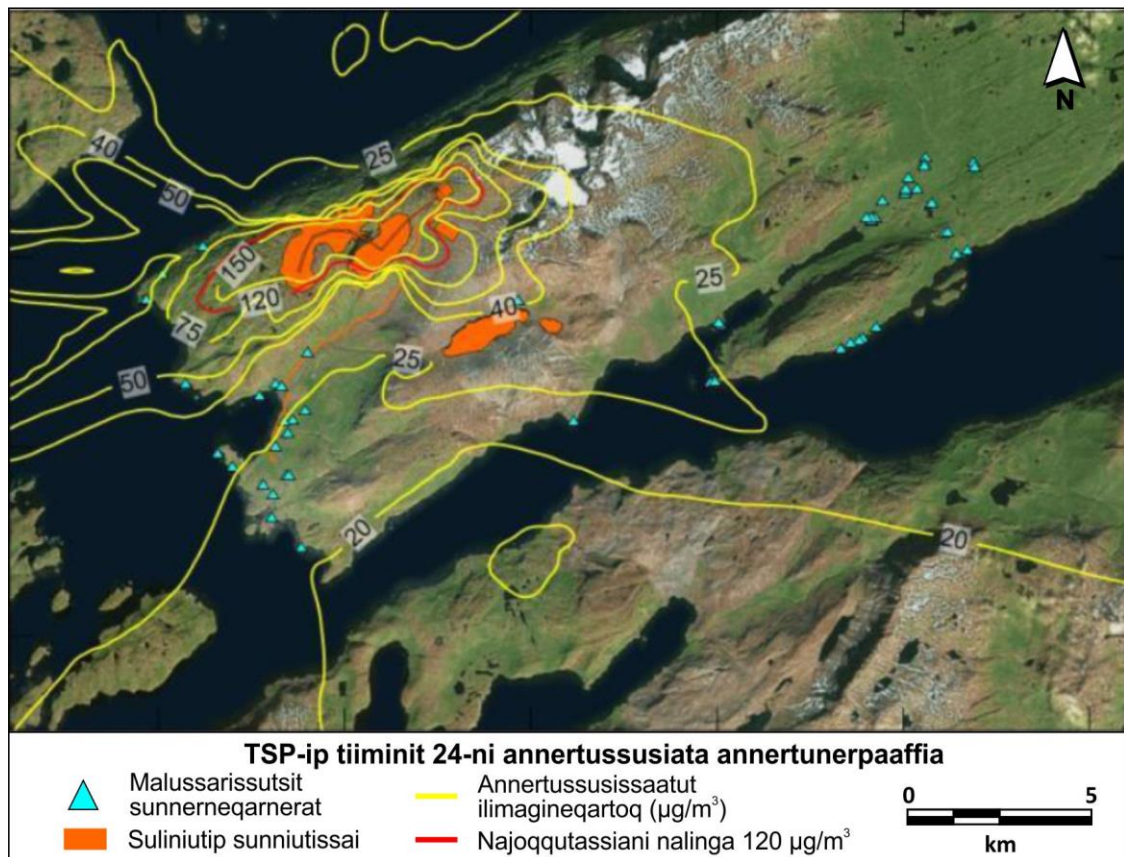
Takussutissiaq 7-5 Pujoralaat ikerinnakkut ingerlasut eqimattat akunnerit 24-it iluanni (tunuliaqutaasut ilanngullugit) (uannga: ERM, 2018)
