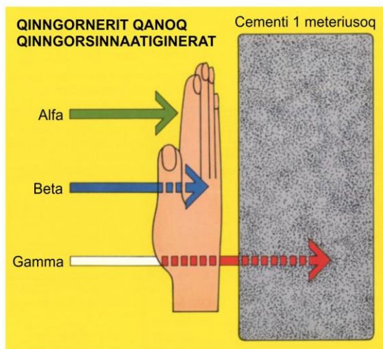
Alfamik, betamik gammamillu qinngornerit timimut pitarsinnaanerannut takussutissiaq (Najoqqutaq: Arcadis, 2015).
