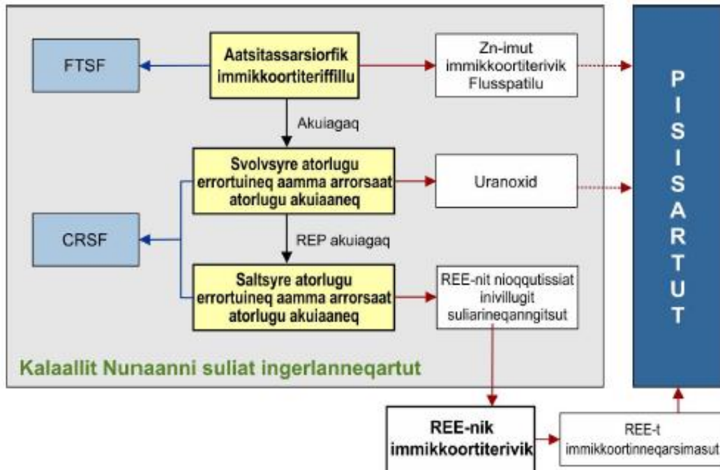
Takussutissiaq 3-4 Suliffissuarmi suliaqarnerup ingerlanera diagraminngorlugu
