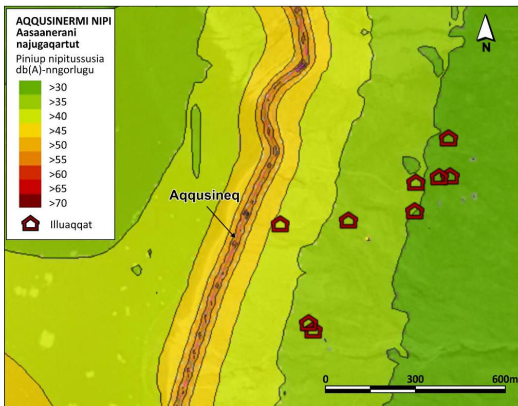
Takussutissiaq 7-6 Nipiliornerup annertussusia aqqusinnermi isaaffiusumi illuaqqat aasarsiortarfiit eqqaanniittumi (uannga: Orbicon, 2015)
