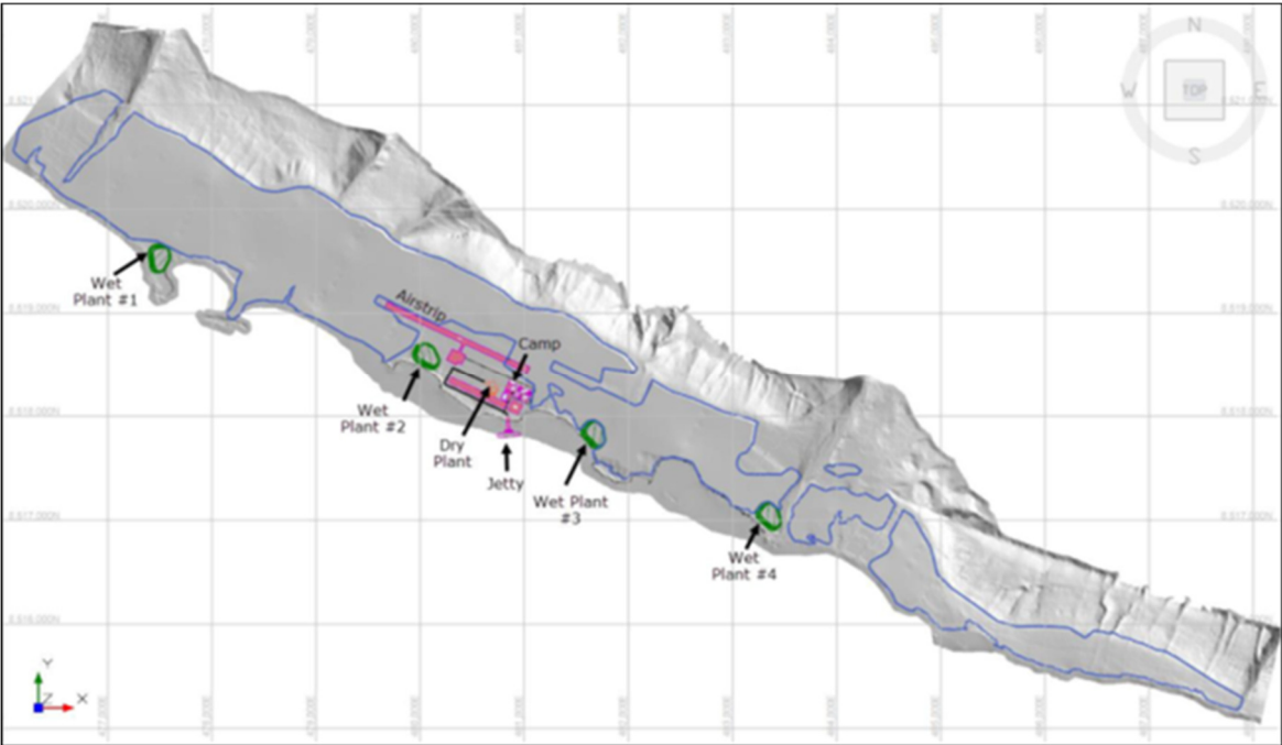
Assiliartaliussaq 3. Aatsitassarsiorfiup aaqqissugaanera, tassaniipput imeq atorlugu akuiaaviup inissiffissai sisamaasut kiisalu najugaqarfimmi ataavartumi imeq atornagu immikkoortiteriviup inissisimaffissaa. Ti-tarnerit tungujortut tassaapput piffiit piiaaffiusussat.
