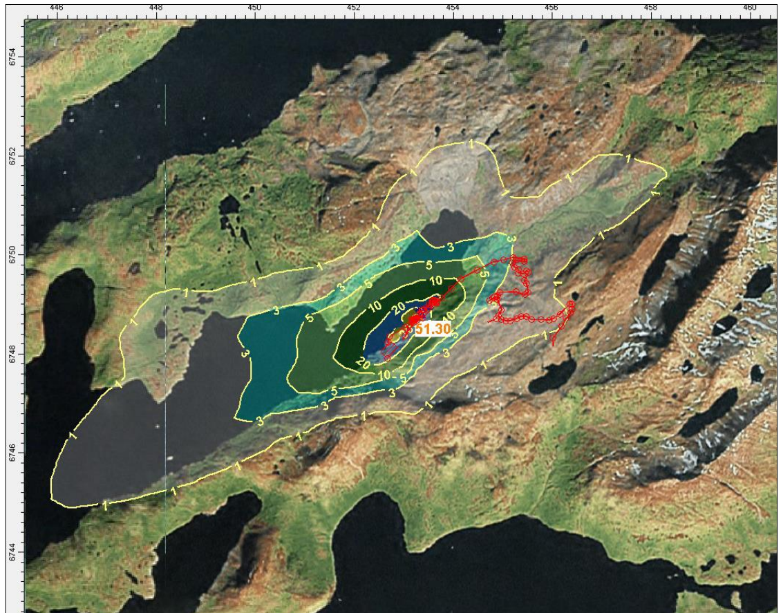
Ass. 9.1 Kangerlummi Piiaaffimmut atatillugu nunap assinga Isoliniusoq pujoralammik ukiumut kivorarsimassut kg/ha-nngorlugit. Kivorarsimassutsip annerpaartaa ukiumut 51,30 kg/ha-iusoq nalu-naarsorneqarpoq (imaluunniit ullormut 14 mg/m 2 ).
