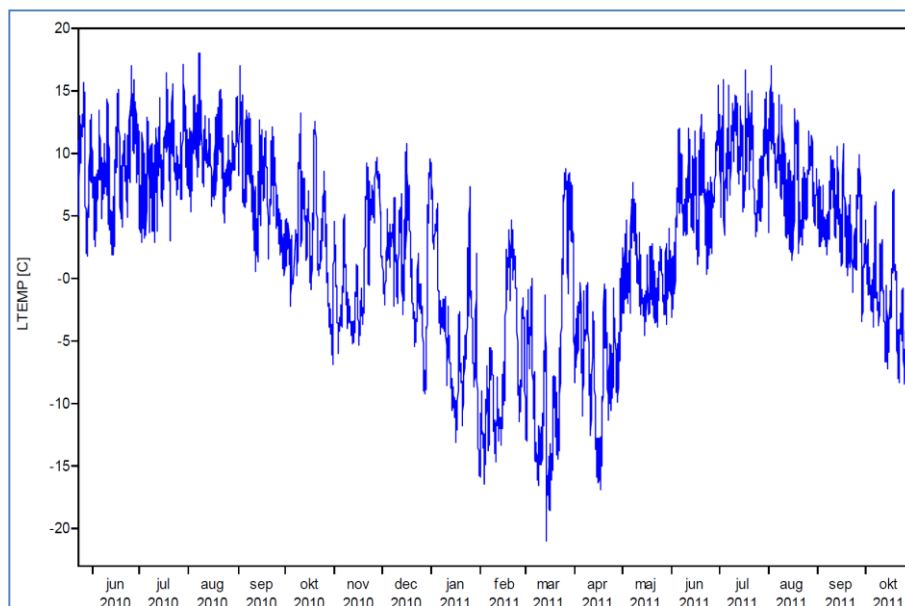
Ass. 6.11 Silap kissassusaa (grad-it centigradillu) Killavaat Alannguani silasiorfimmi Juuni 2010 Oktobarilu 2011 akornanni uuttorneqarsimasoq. Silasiorfik 450 meter-inik qatsitigisumiippoq
